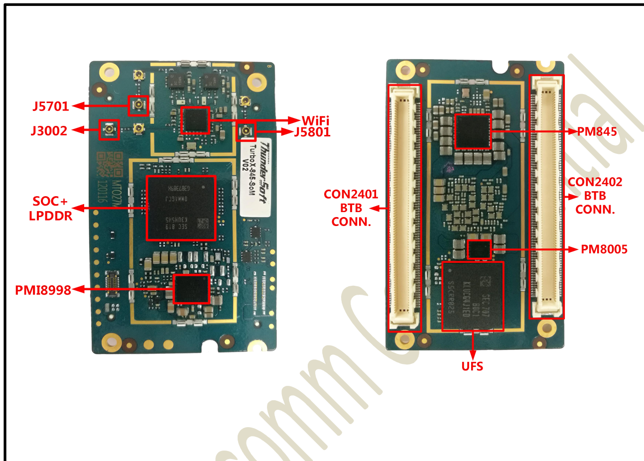
Figure 1.1- 1 TurboX D845 SOM Key component Location
