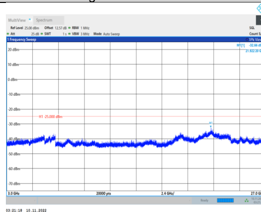
Band41-20MHz-QPSK-41140-1RB#0- Range3:3000~27000MHz
