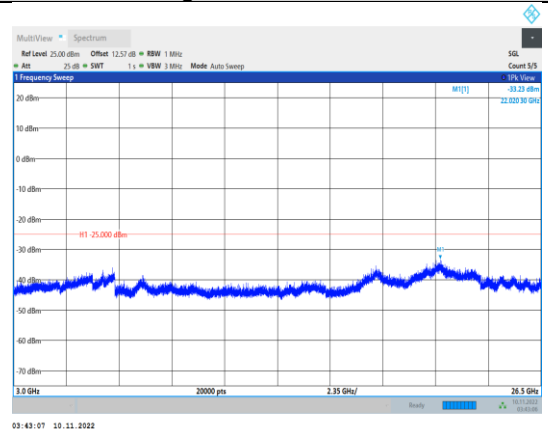
Band38-20MHz-QPSK-37850-1RB#0- Range3:3000~26500MHz
