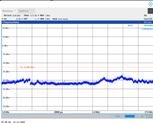
Band41-5MHz-QPSK-41215-1RB#0- Range3:3000~27000MHz
