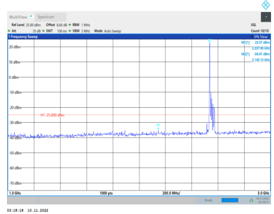
Band41-20MHz-QPSK-40140-1RB#0- Range2:1000~3000MHz
