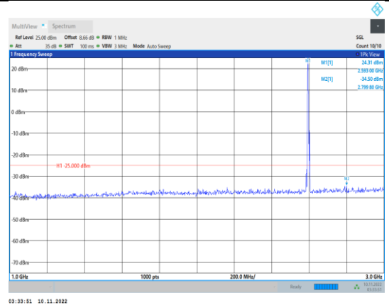
Band41-5MHz-QPSK-40640-1RB#0- Range2:1000~3000MHz
