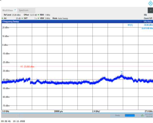
Band41-5MHz-QPSK-40065-1RB#0- Range3:3000~27000MHz
