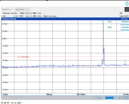
Band41-10MHz-QPSK-40640-1RB#0- Range2:1000~3000MHz
