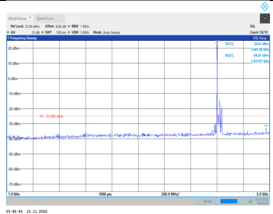
Band38-20MHz-QPSK-38150-1RB#0- Range2:1000~3000MHz
