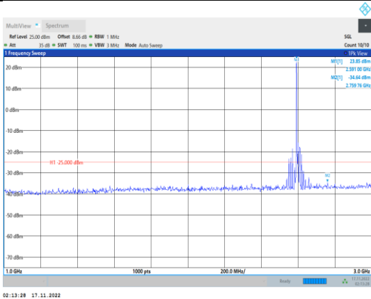
Band41-10MHz-64QAM-40640-1RB#0- Range2:1000~3000MHz
