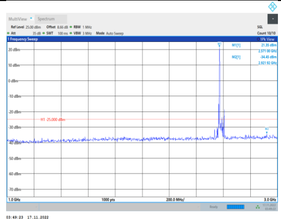
Band38-20MHz-64QAM-37850-1RB#0- Range2:1000~3000MHz
