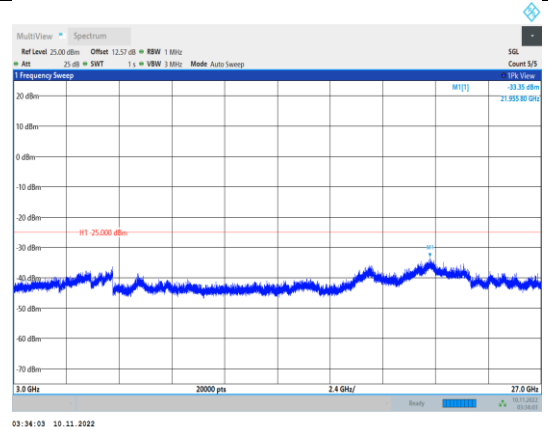
Band41-5MHz-QPSK-40640-1RB#0- Range3:3000~27000MHz
