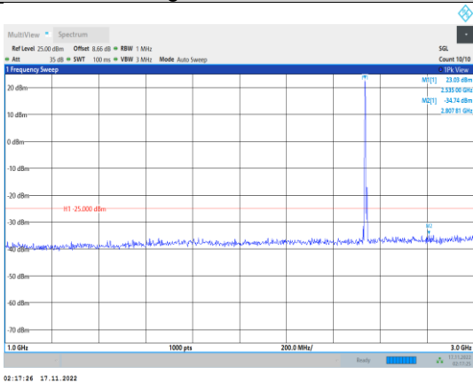
Band41-5MHz-64QAM-40065-1RB#0- Range2:1000~3000MHz
