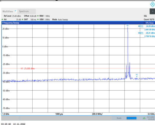
Band41-15MHz-QPSK-41165-1RB#0- Range2:1000~3000MHz
