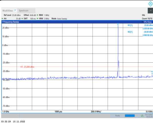
Band41-5MHz-QPSK-40065-1RB#0- Range2:1000~3000MHz
