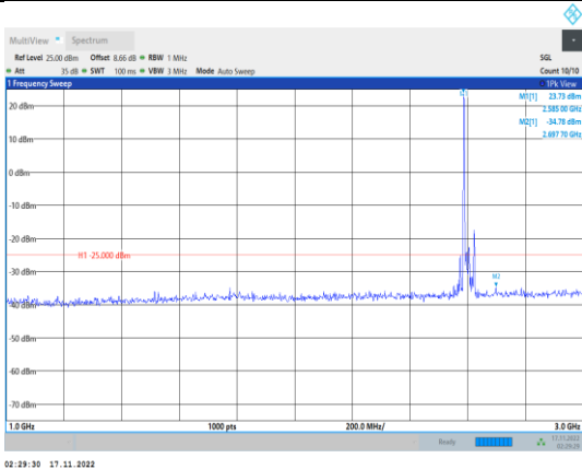
Band41-20MHz-64QAM-40640-1RB#0- Range2:1000~3000MHz
