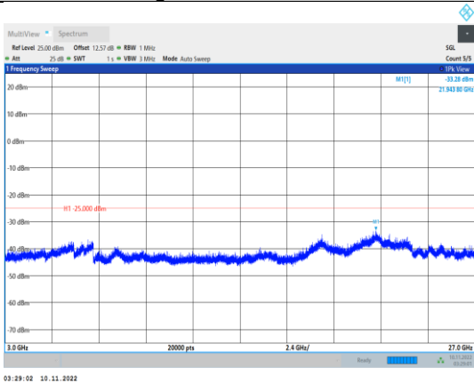
Band41-10MHz-QPSK-40640-1RB#0- Range3:3000~27000MHz
