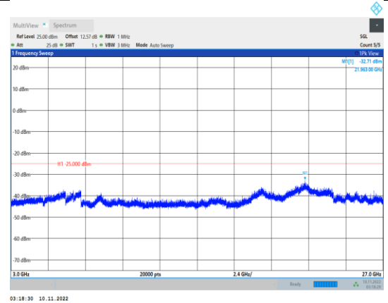
Band41-20MHz-QPSK-40140-1RB#0- Range3:3000~27000MHz
