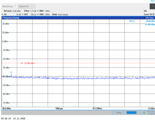
Band41-5MHz-QPSK-40065-1RB#0- Range1:30~1000MHz
