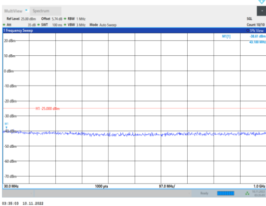
Band41-5MHz-QPSK-41215-1RB#0- Range1:30~1000MHz
