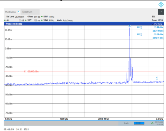
Band38-20MHz-QPSK-37850-1RB#0- Range2:1000~3000MHz
