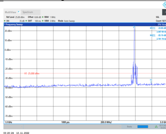
Band41-20MHz-16QAM-40640-1RB#0- Range2:1000~3000MHz
