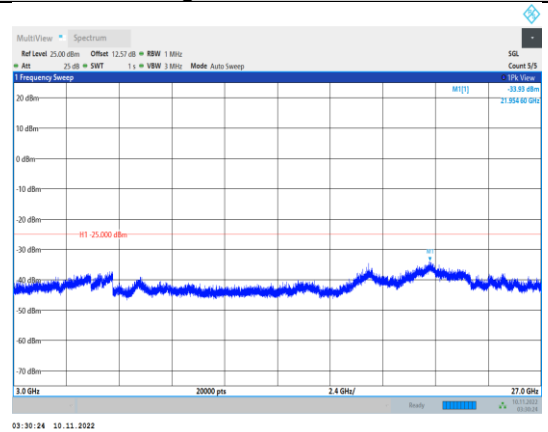
Band41-10MHz-QPSK-41190-1RB#0- Range3:3000~27000MHz
