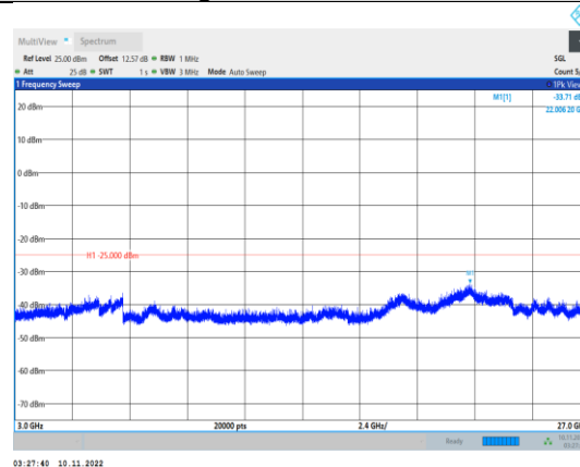
Band41-10MHz-QPSK-40090-1RB#0- Range3:3000~27000MHz
