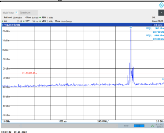
Band41-20MHz-QPSK-40640-1RB#0- Range2:1000~3000MHz
