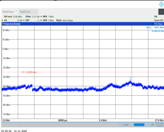
Band41-15MHz-QPSK-41165-1RB#0- Range3:3000~27000MHz
