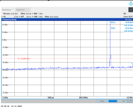
Band41-5MHz-QPSK-41215-1RB#0- Range2:1000~3000MHz
