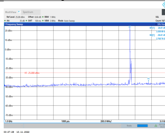
Band41-10MHz-QPSK-40090-1RB#0- Range2:1000~3000MHz
