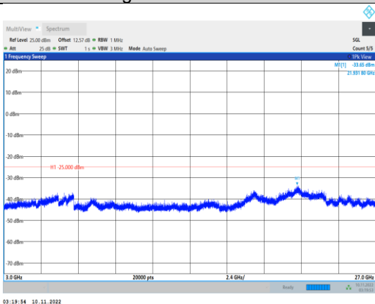
Band41-20MHz-QPSK-40640-1RB#0- Range3:3000~27000MHz
