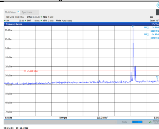
Band41-20MHz-QPSK-41140-1RB#0- Range2:1000~3000MHz
