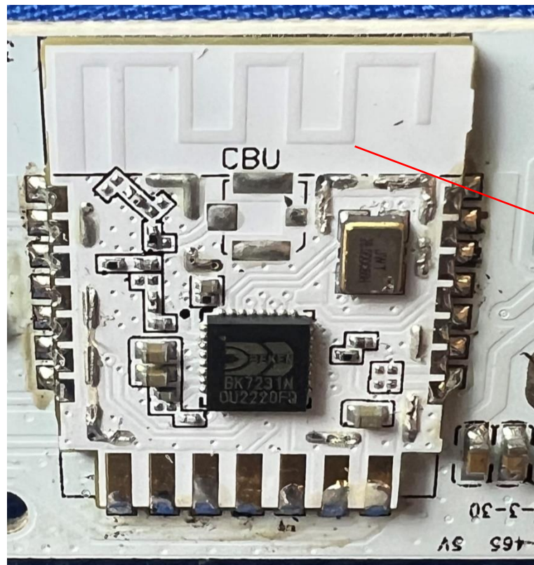
Antenna
