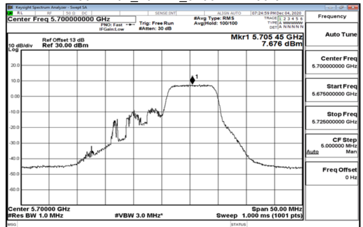
802.11ax_20MHz_5700MHz-26-8
