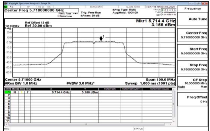
802.11n_40MHz_5710MHz_UNII 3
