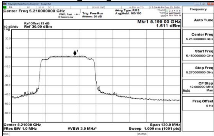
802.11ax_80MHz_5210MHz-484-65
