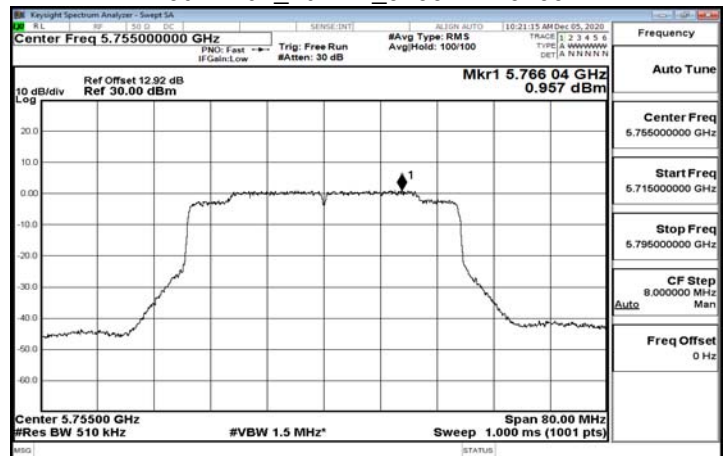
802.11ax_40MHz_5755MHz-242-61
