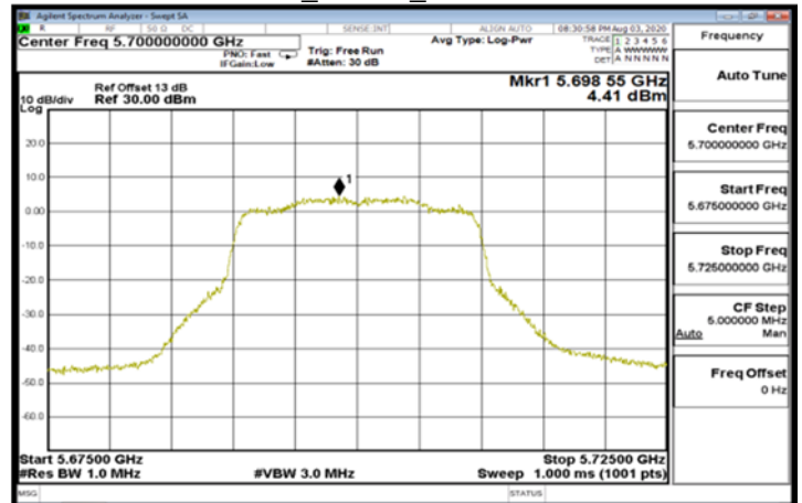
802.11ax_20MHz_5700MHz-106-54
