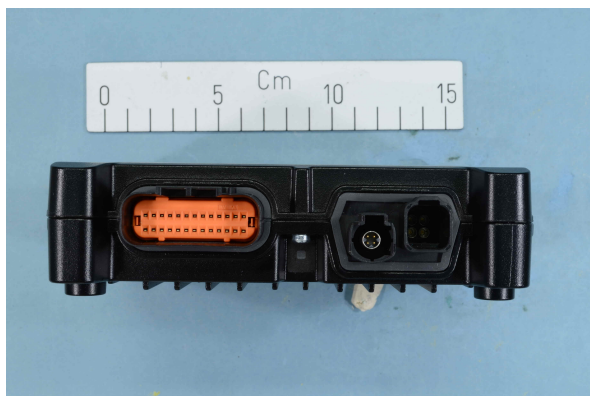
EUT Connectors
