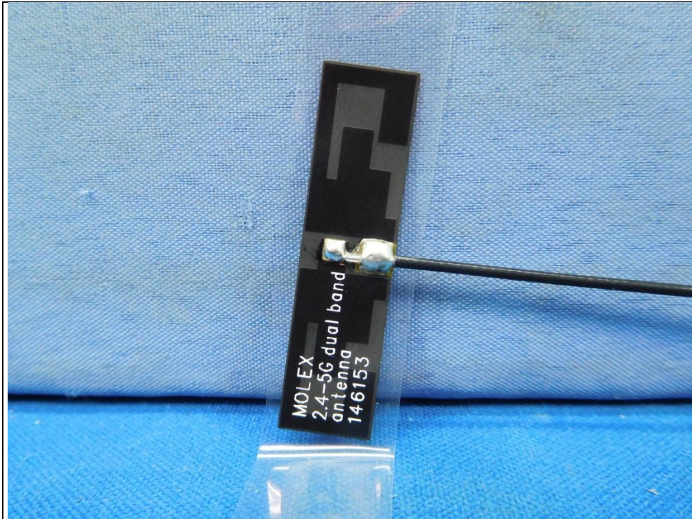
Antenna 11 (Brand: MOLEX ; Model: 1461530150)
