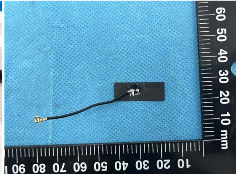
BLE/WiFi Antenna
