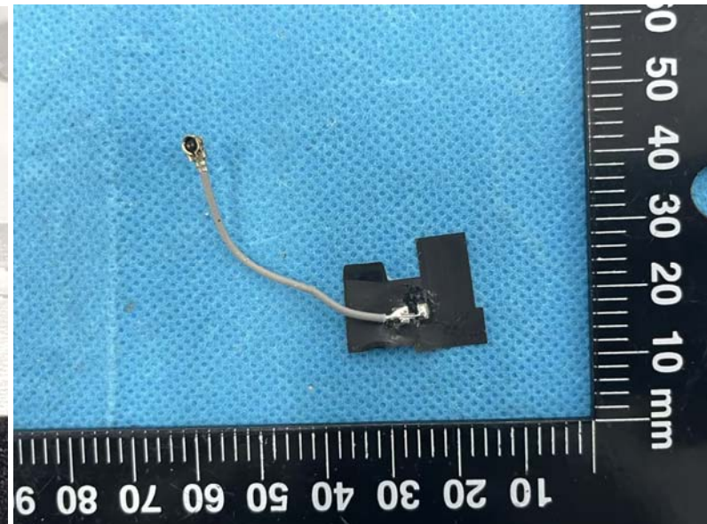
BLE/WiFi Antenna
