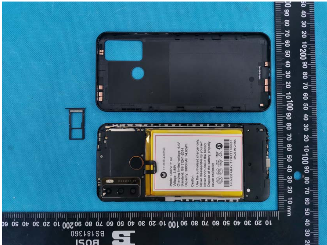
GSM1900/WCDMA B2&B4/LTE B2&B4&B41&B66 Antenna
