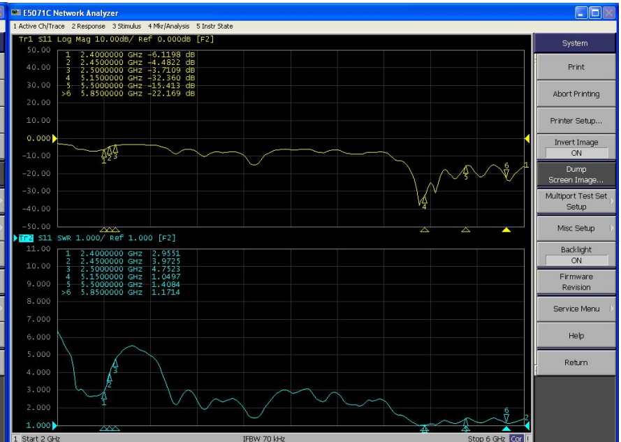
ANT1-5G
