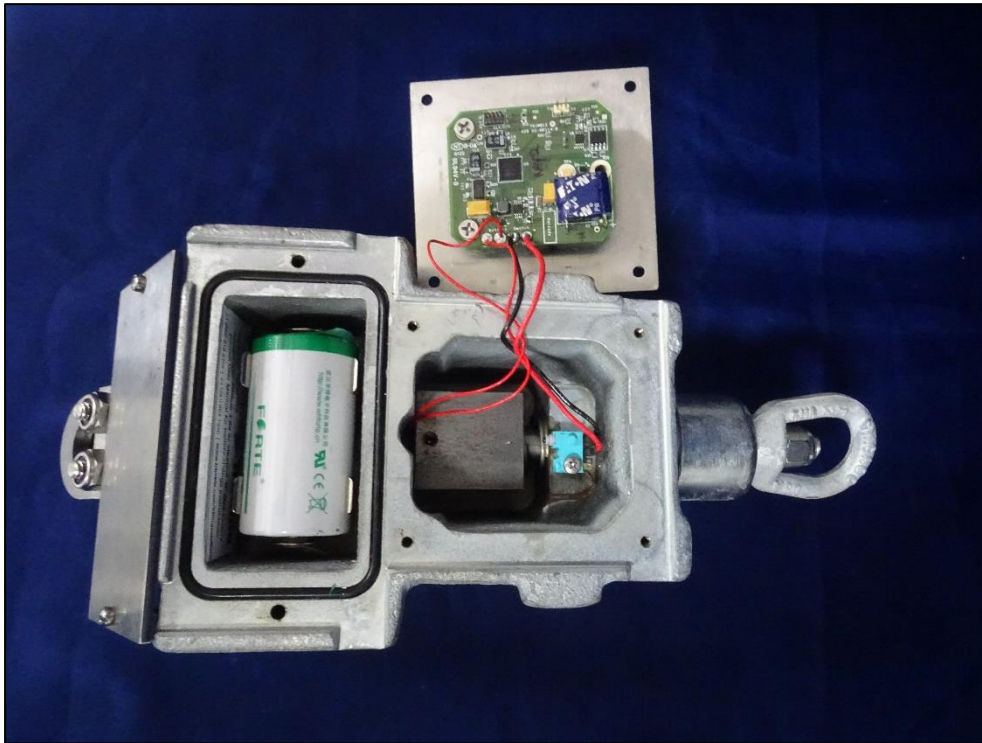
EUT Encloser Open
