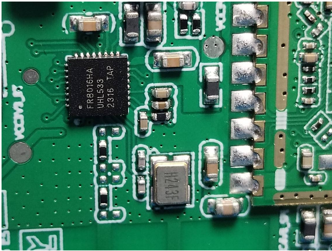
BT ANT
