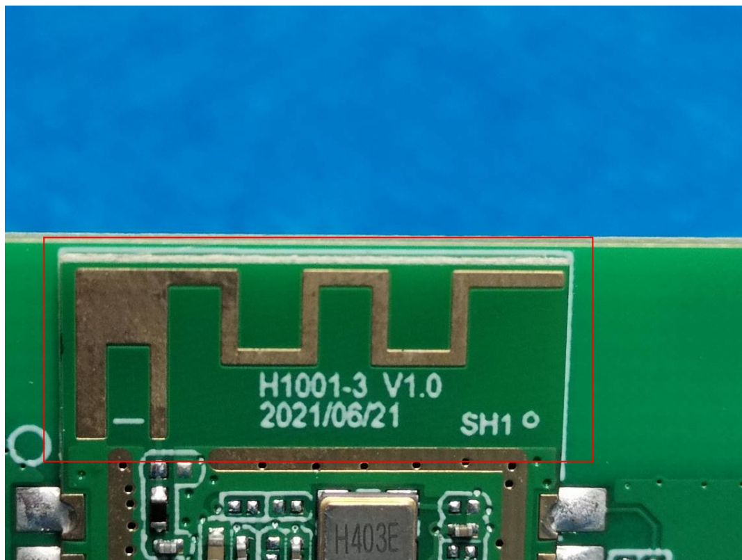
Wi-Fi ANT
