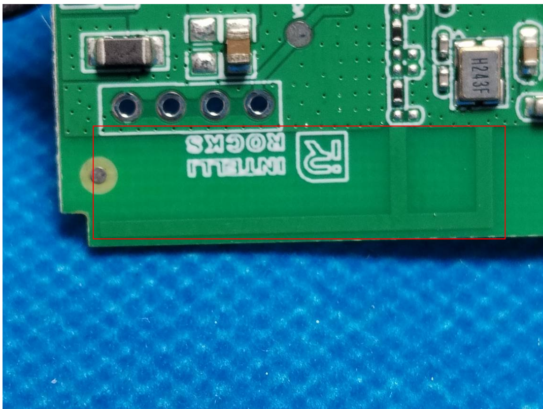
BT ANT
