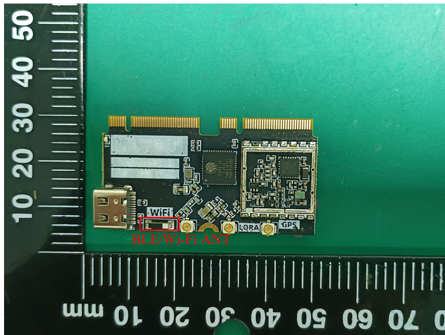
T-BEAM-S3
