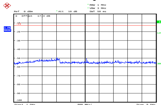
GSM 850 CH-High 1GHz ~ 9GHz
