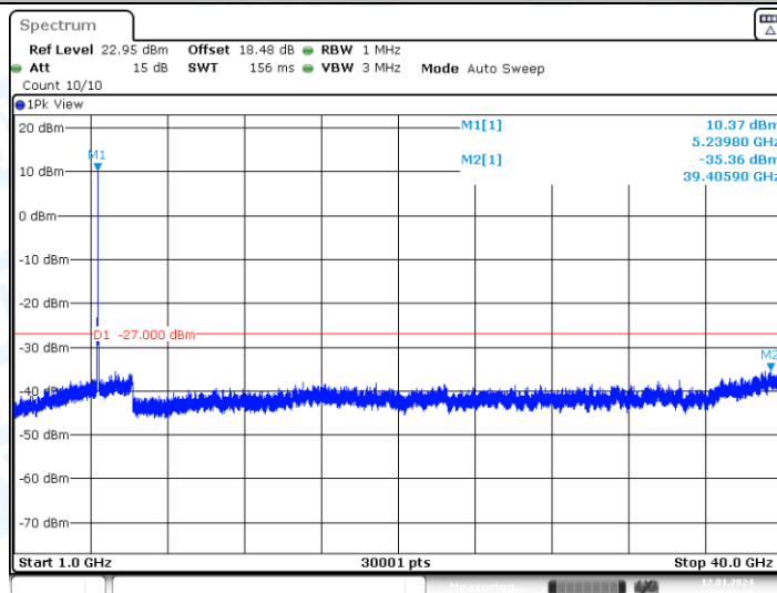
11AX20-CDD_Ant1_5240_1000~40000
