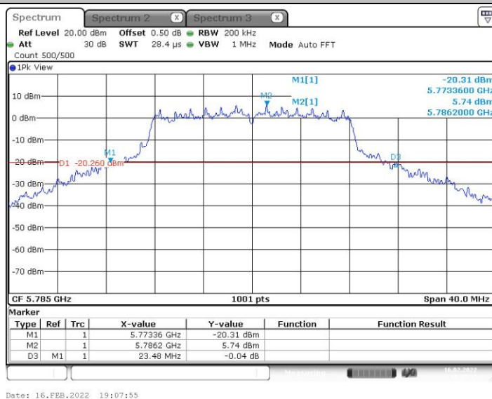
11A_Ant9_5785
