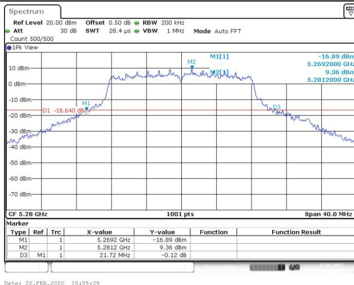
11A_Ant9_5280
