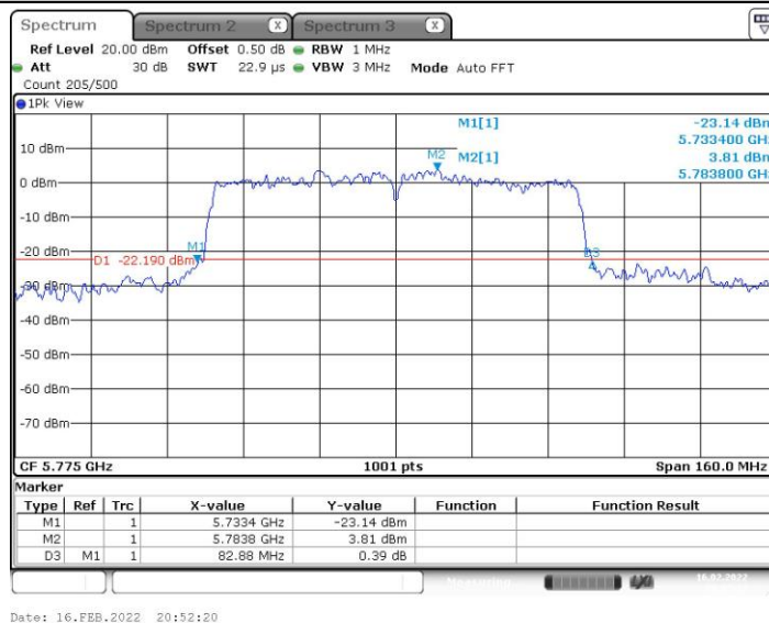
11AC80MIMO_Ant8_5775
