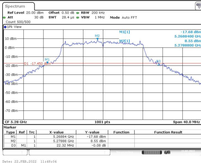
11A_Ant9_5280
