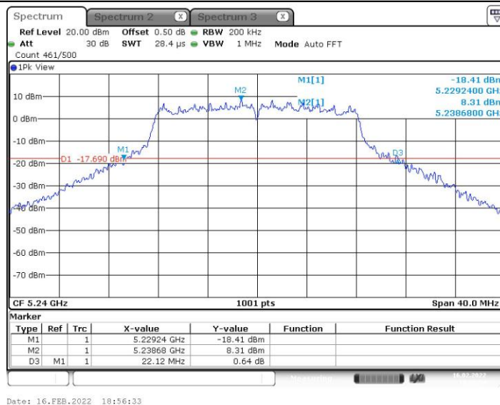
11A_Ant8_5240
