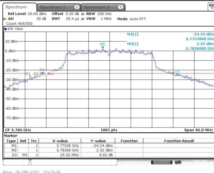
11A_Ant9_5785
