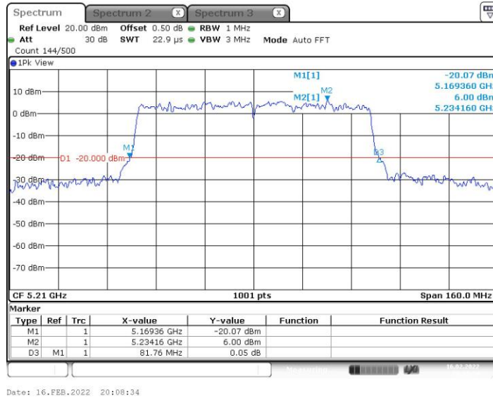
11AC80MIMO_Ant9_5210
