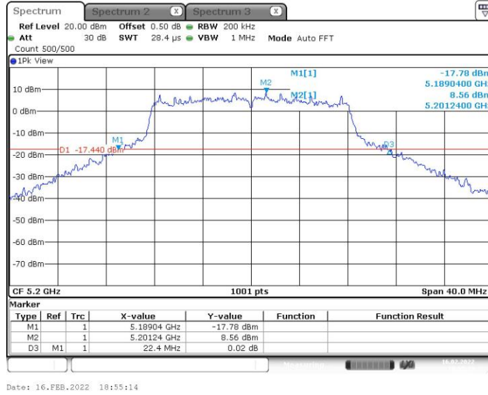
11A_Ant9_5200
