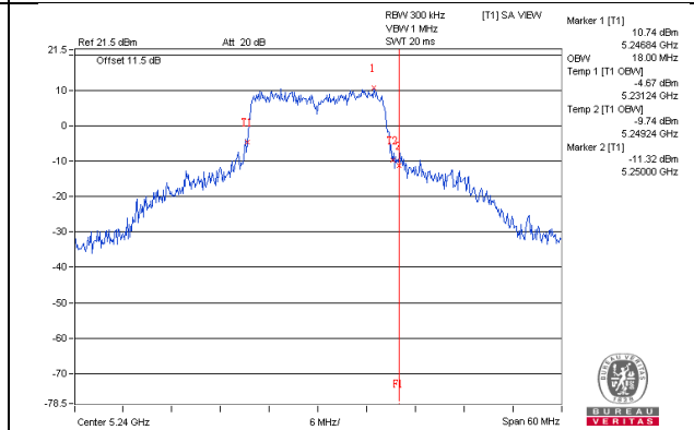
802.11ac(VHT20)_Chain1 / CH48
