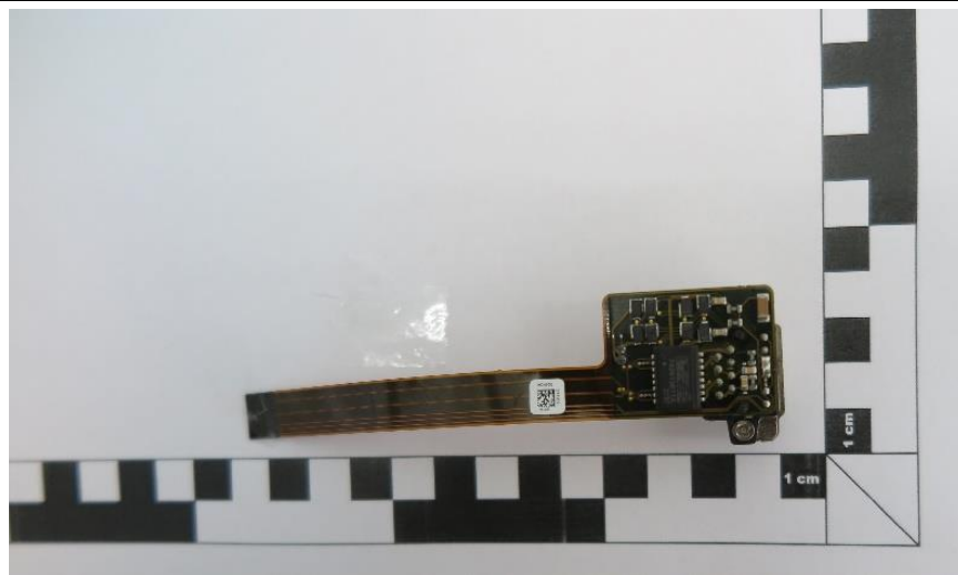
PCB 6 BOTTOM
