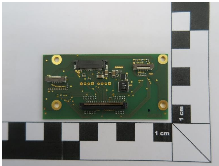
PCB 2 TOP
