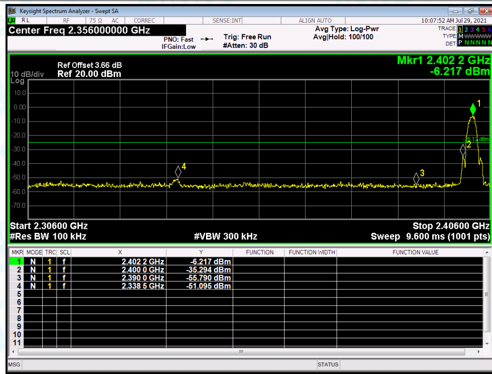
Band Edge NVNT BLE 2Mbps 2402MHz Ant1 Emission
