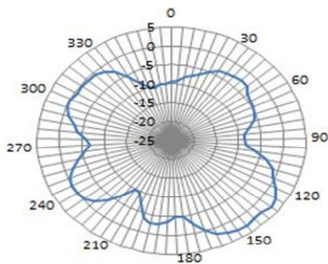
XZ-2450MHz
