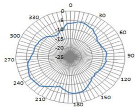
YZ-2450MHz
