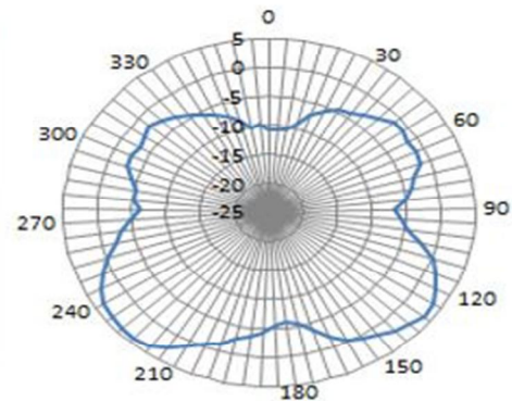
YZ-2450MHz
