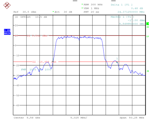
802.11ac20_5580MHz_Chain 1
