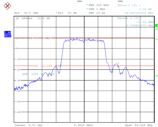
802.11ac20 5720MHz Chain 1
