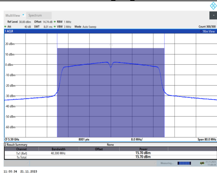
11N40MIMO_Ant2_5590
