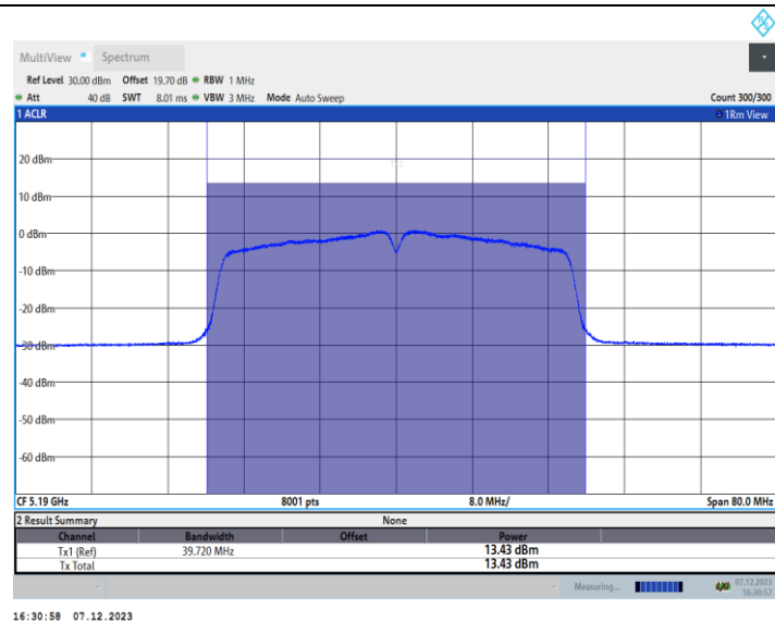
11AC40MIMO_Ant2_5190
