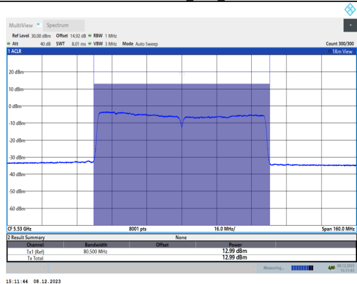
11AC80MIMO_Ant2_5530
