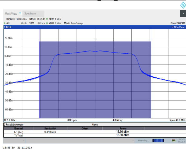
11AC20MIMO_Ant2_5600
