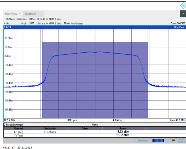
11AX20MIMO_Ant2_5200
