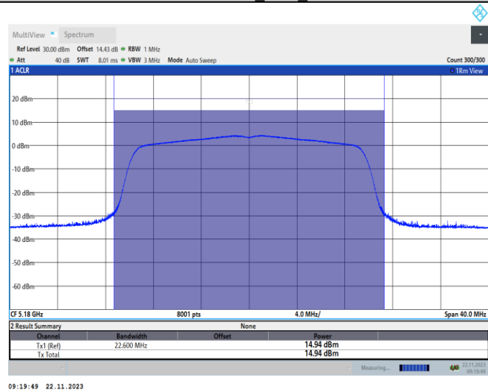
11AX20MIMO_Ant2_5180
