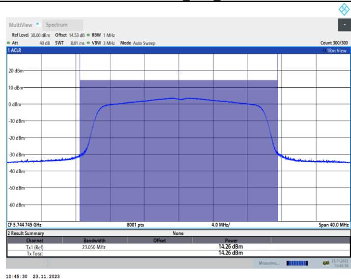
11AX20MIMO_Ant2_5745
