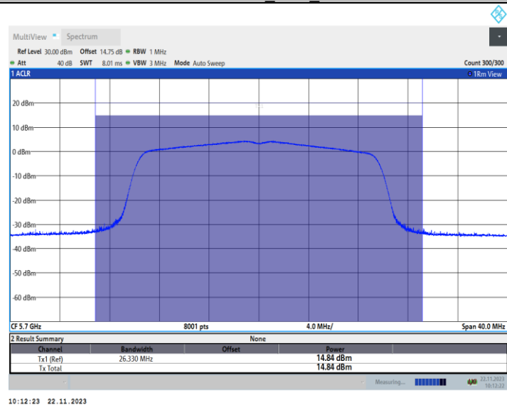
11AX20MIMO_Ant2_5700
