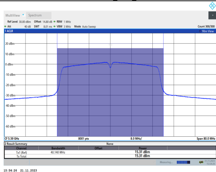
11AC40MIMO_Ant2_5590
