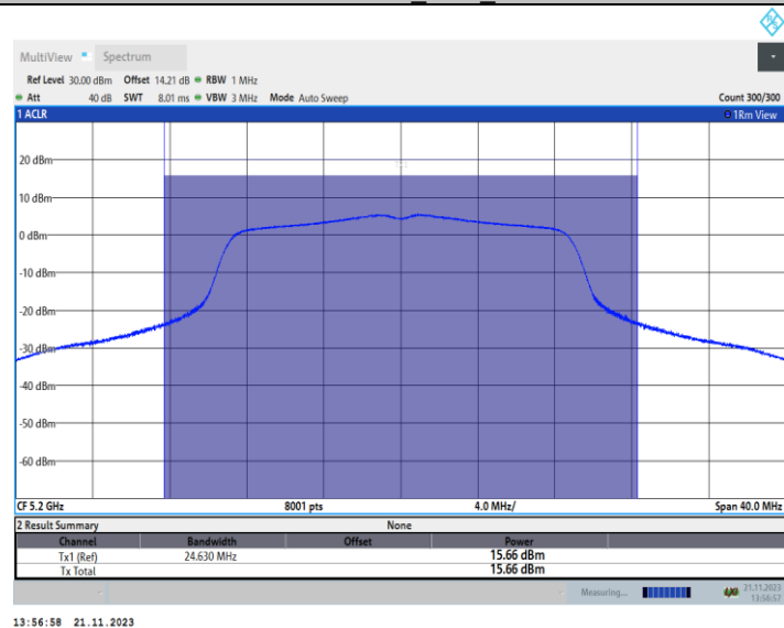
11AC20MIMO_Ant2_5200
