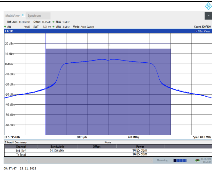
11AC20MIMO_Ant2_5745
