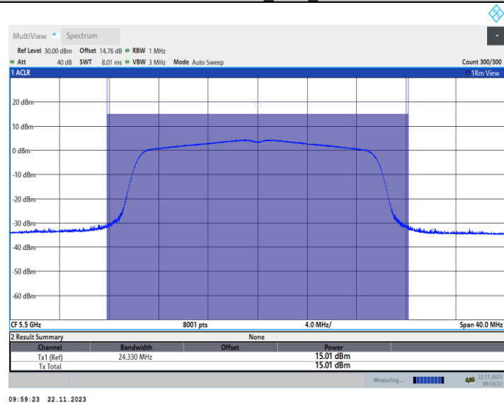
11AX20MIMO_Ant2_5500
