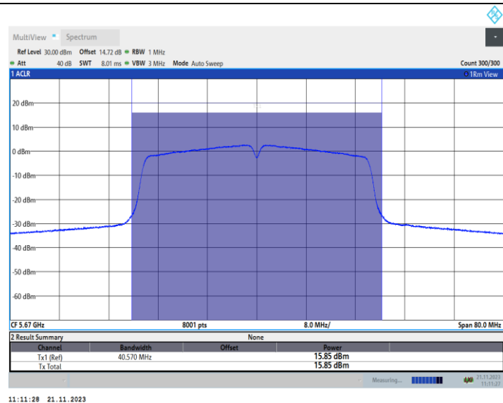
11N40MIMO_Ant2_5670
