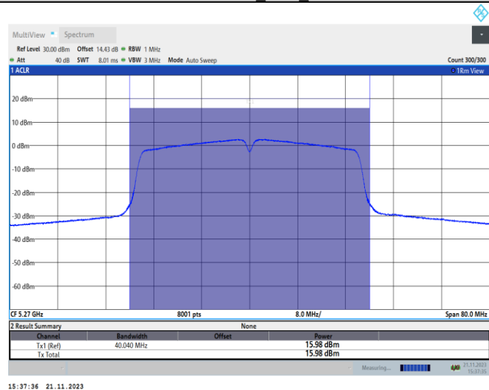
11AC40MIMO_Ant2_5270
