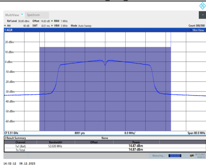
11N40MIMO_Ant2_5510
