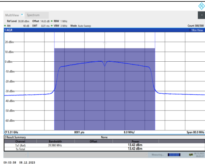
11N40MIMO_Ant2_5310
