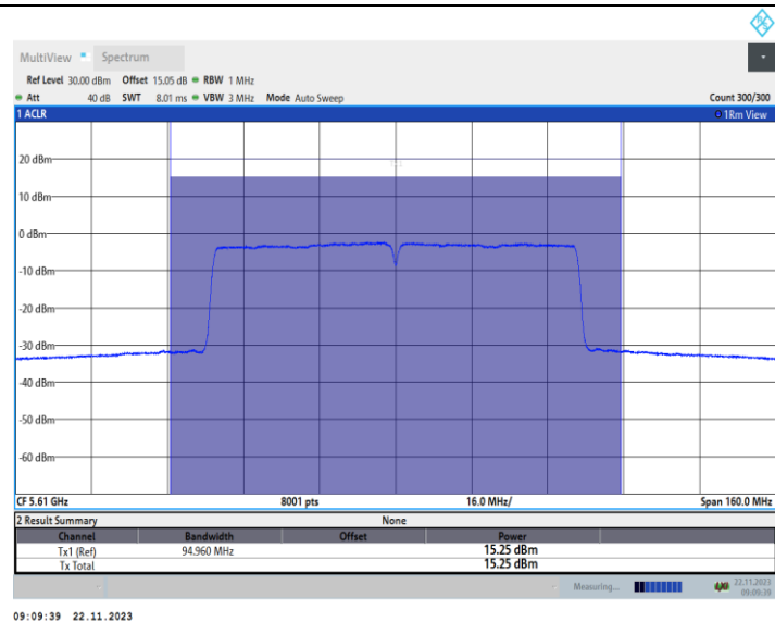
11AC80MIMO_Ant2_5610
