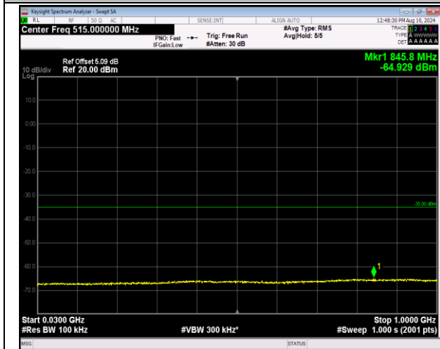
7-7-10MHz-20MHz-QPSK-QPSK-21006-21150-50RB#0-1 00RB#0-30~1000MHz-PASS
