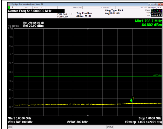
7-7-10MHz-20MHz-QPSK-QPSK-21206-21350-50RB#0-100RB#0-30~1000MHz-PASS
