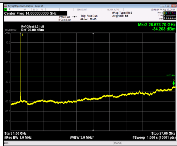
7-7-10MHz-20MHz-QPSK-QPSK-20805-20949-1RB#49-0R B#0-1000~27000MHz-PASS
