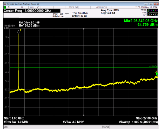
7-7-10MHz-20MHz-QPSK-QPSK-21206-21350-1RB#0-1RB #99-1000~27000MHz-PASS
