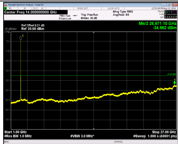
7-7-10MHz-20MHz-QPSK-QPSK-21206-21350-50RB#0-100RB#0-1000~27000MHz-PASS
