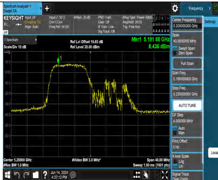
11BE20MIMO Ant4 5200 26Tone RU0
