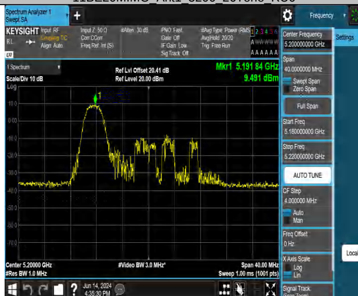
11BE20MIMO Ant1 5200 106Tone RU53
