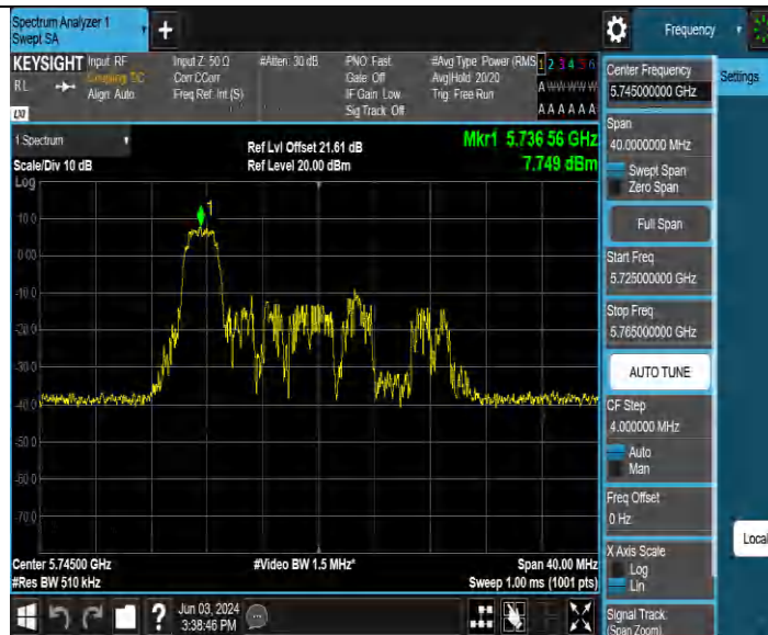
11BE20MIMO Ant1 5745 106Tone RU53
