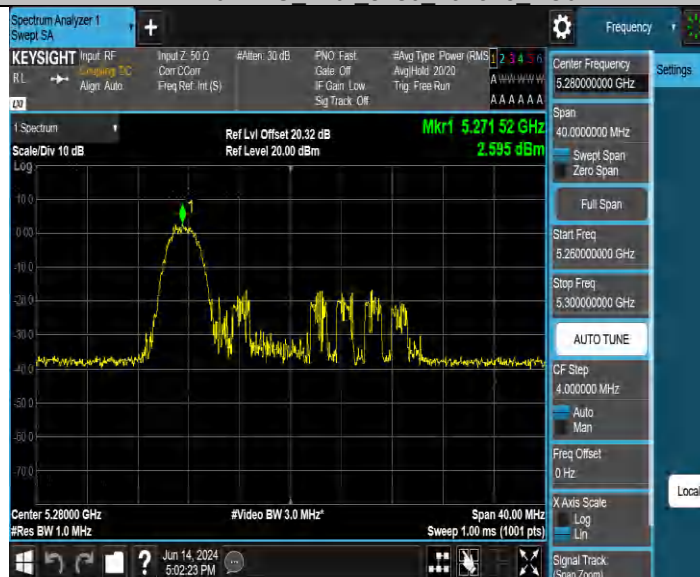
11BE20MIMO Ant4 5280 106Tone RU53
