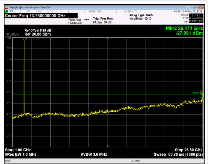
Band38-20MHz-QPSK-38000-1RB#0-Range2:1000~2 6500MHz
