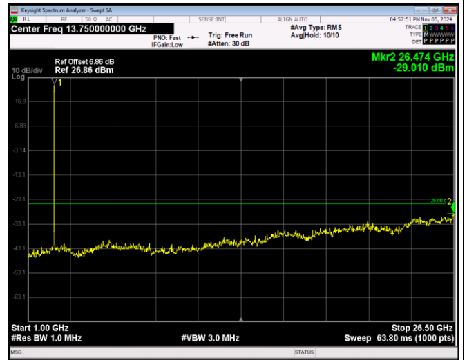
Band38-5MHz-QPSK-38000-1RB#0-Range2:1000~26 500MHz
