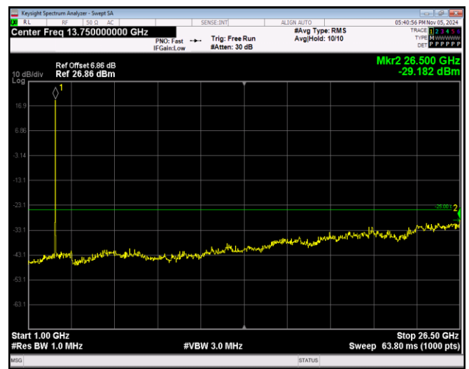
Band41-5MHz-QPSK-40065-1RB#0-Range2:1000~26500MHz
