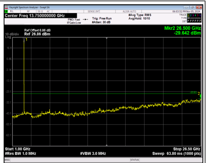
Band41-5MHz-QPSK-41215-1RB#0-Range2:1000~26 500MHz
