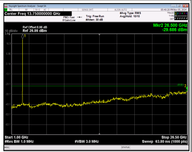
Band38-20MHz-QPSK-38150-1RB#0-Range2:1000~2 6500MHz
