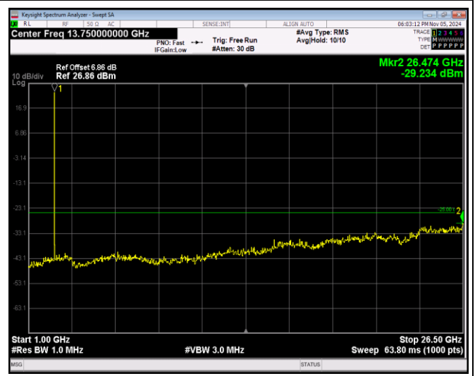
Band41-5MHz-16QAM-40065-1RB#0-Range2:1000~2 6500MHz
