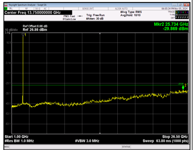
Band41-5MHz-16QAM-40065-1RB#0-Range2:1000~2 6500MHz
