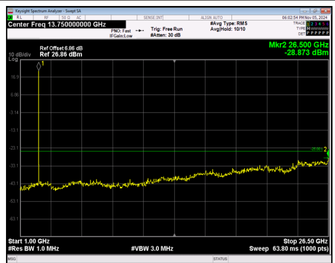
Band41-5MHz-QPSK-40640-1RB#0-Range2:1000~26500MHz
