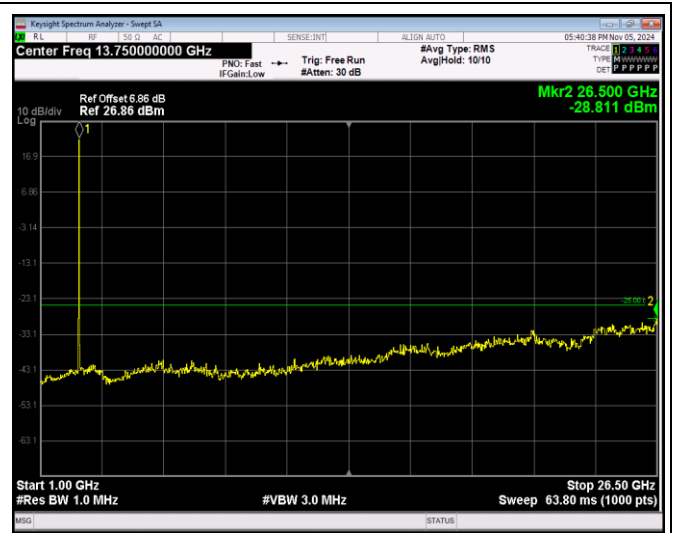
Band38-20MHz-64QAM-37850-1RB#0-Range2:1000~26500MHz
