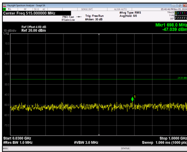
Band41-5MHz-QPSK-40065-1RB#0-Range1:30~1000MHz
