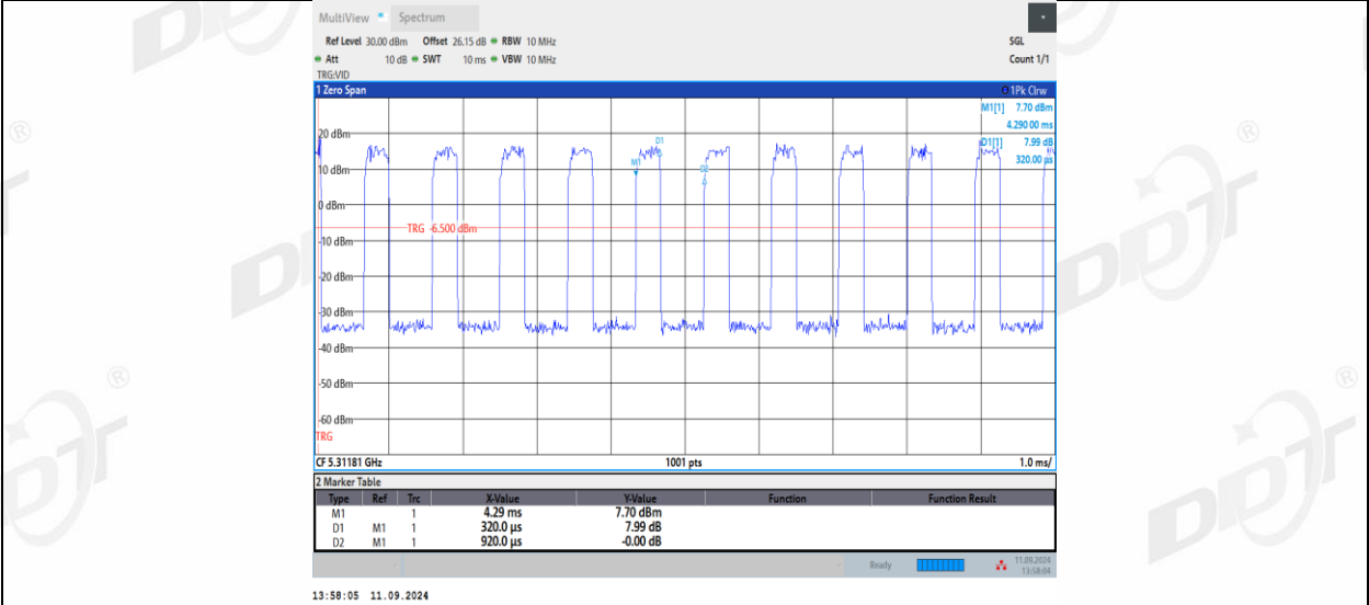
11AX20MIMO_Ant1_5320_52Tone_RU39
