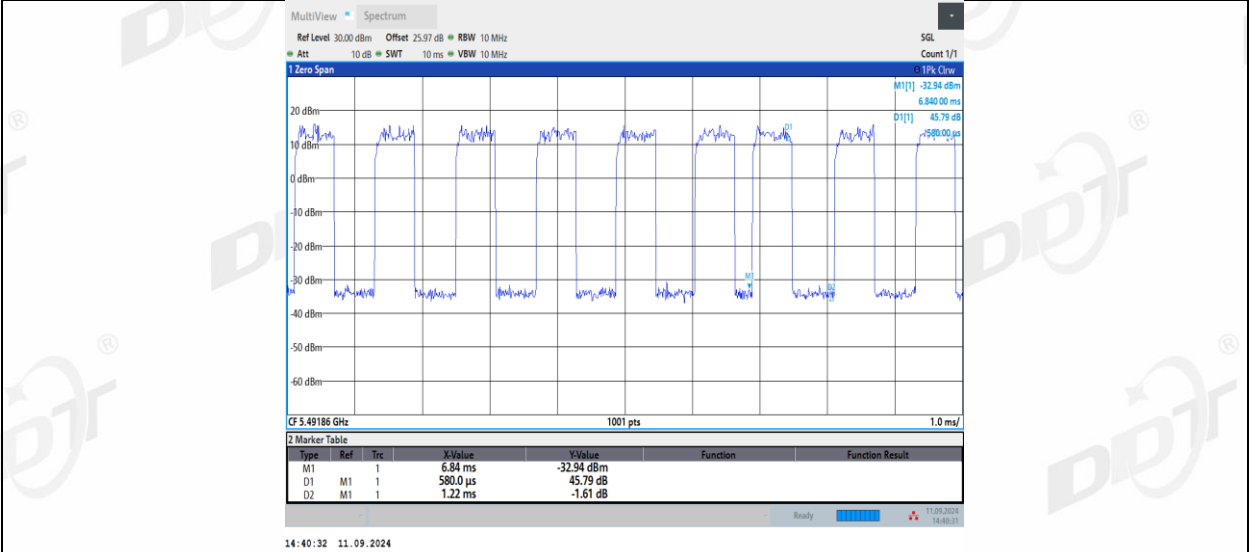
11AX20MIMO_Ant2_5500_26Tone_RU4
