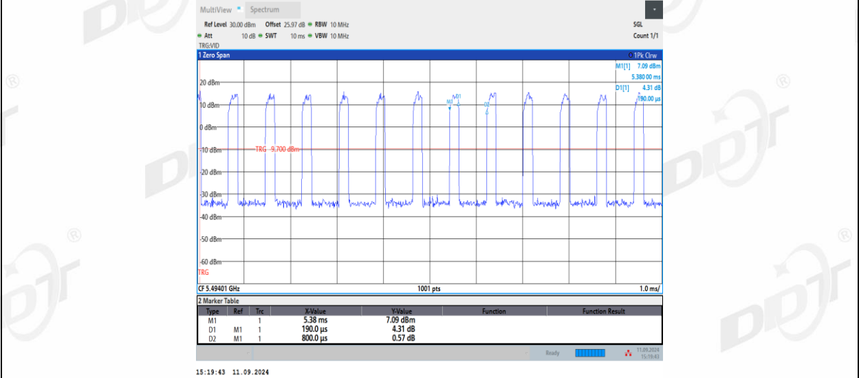
11AX20MIMO_Ant2_5500_106Tone_RU54
