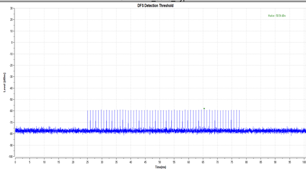
40MHz BW_5510_Type2
