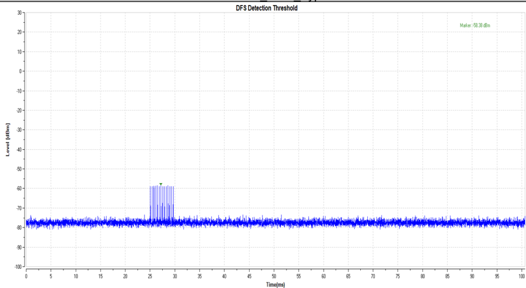
40MHz BW_5510_Type5
