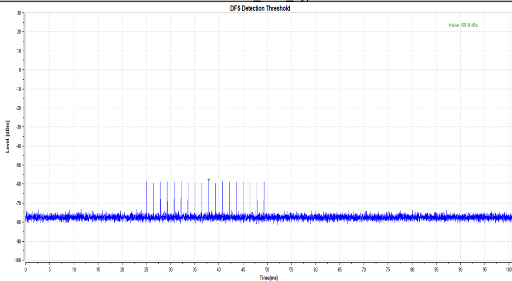
40MHz BW_5510_Type1
