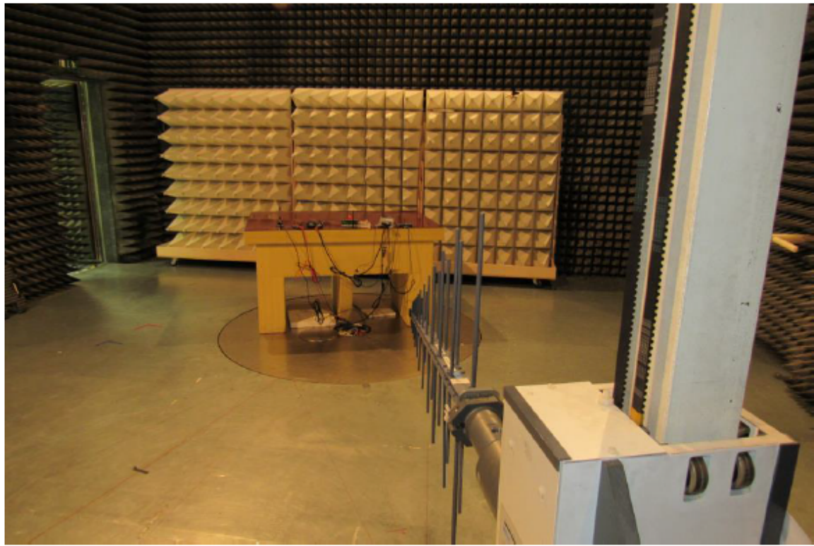
FCC part 24E - Testsetup
