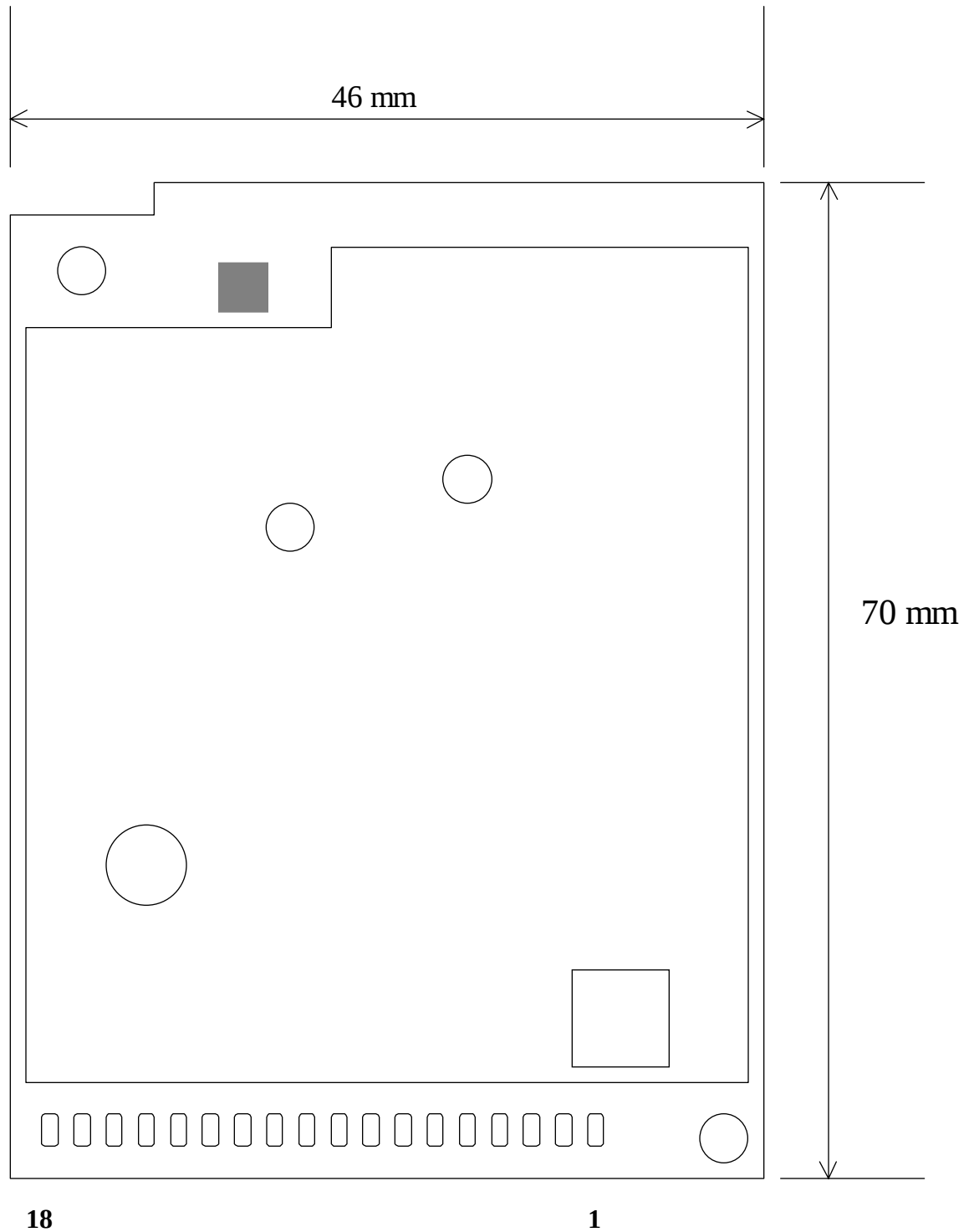
900 MHz RF Module Dimensions
