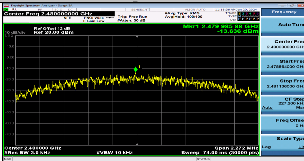
BLE_2M-Ant1-2480
