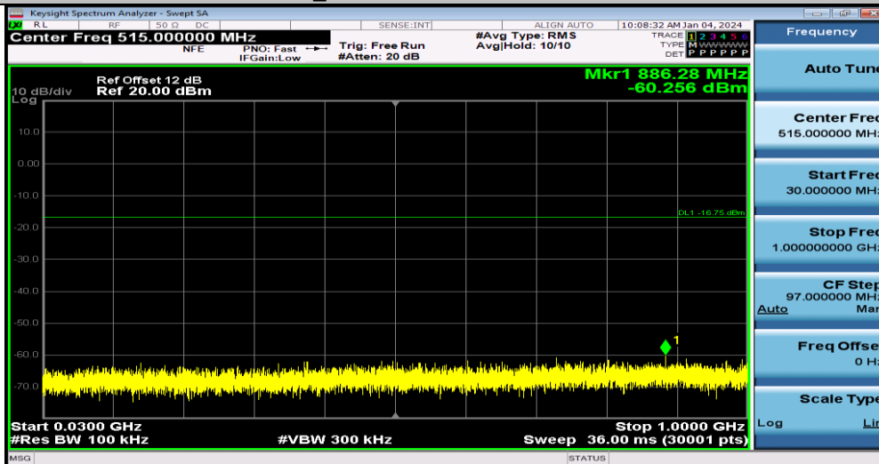
BLE_2M-Ant1-2480-30~1000
