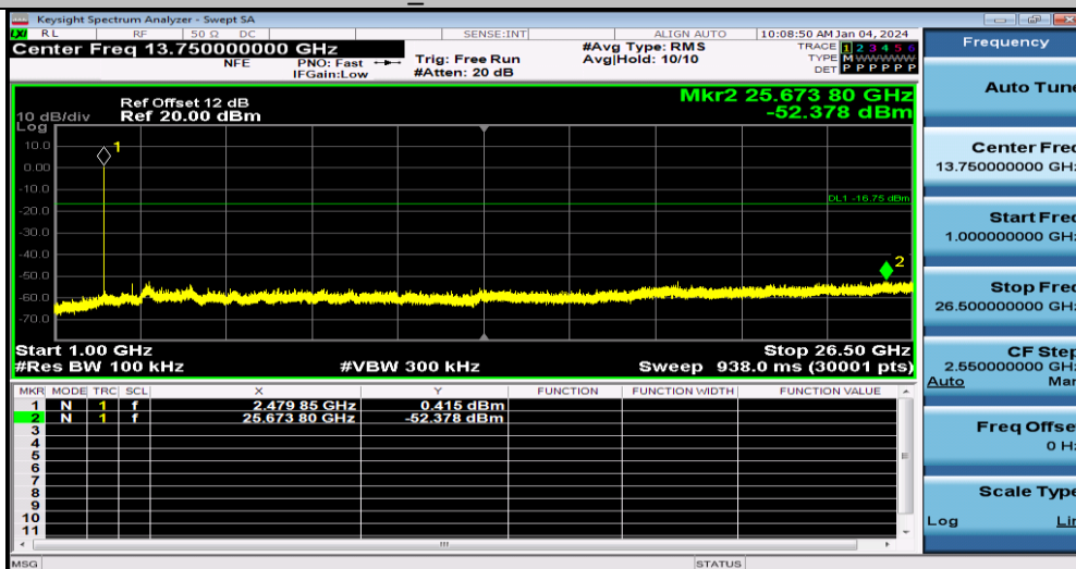
BLE_2M-Ant1-2480-1000~26500
