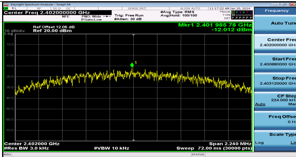
BLE_2M-Ant1-2402
