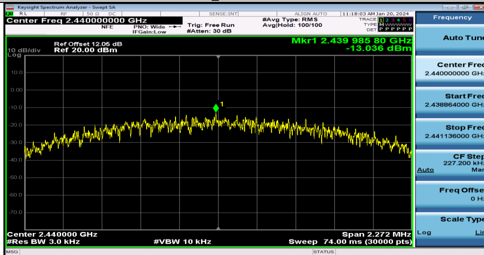
BLE_2M-Ant1-2440
