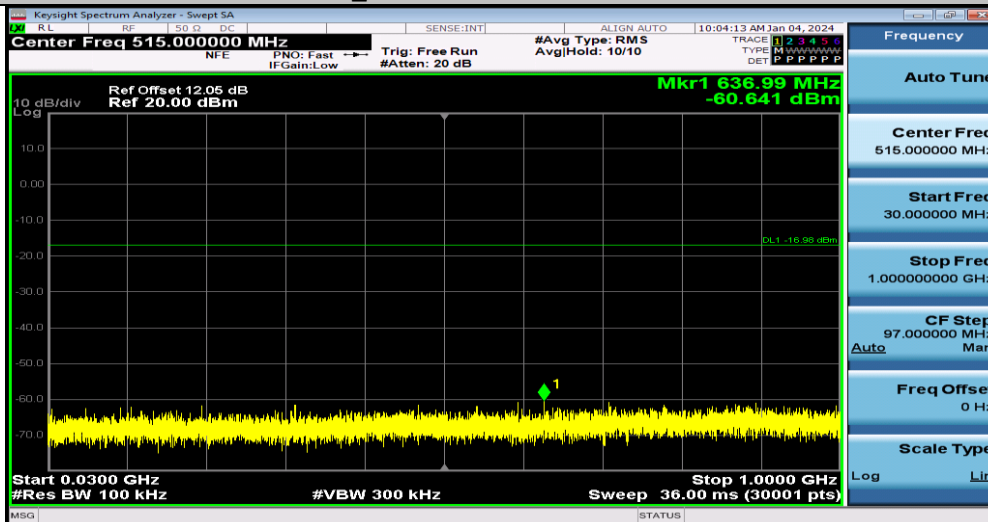
BLE_2M-Ant1-2440-30~1000
