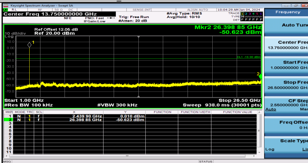
BLE_2M-Ant1-2440-1000~26500
