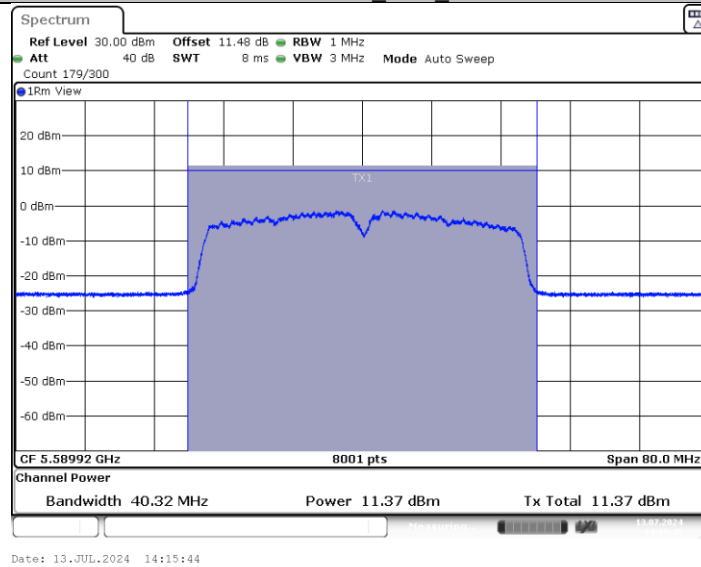
11AC40MIMO_Ant2_5590
