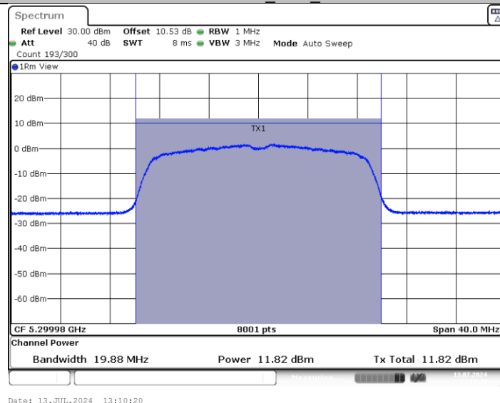
11AC20MIMO_Ant2_5300
