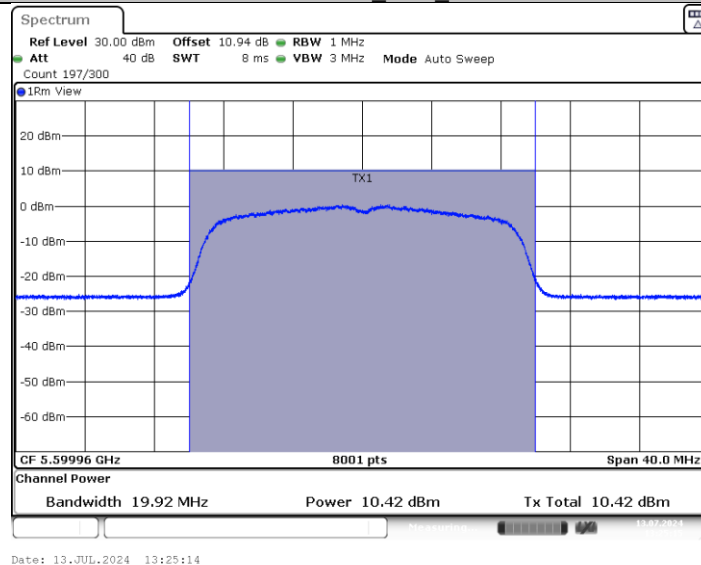
11AC20MIMO_Ant2_5600
