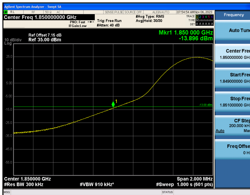
Band2-15MHz-16QAM-18675-1RB#74
