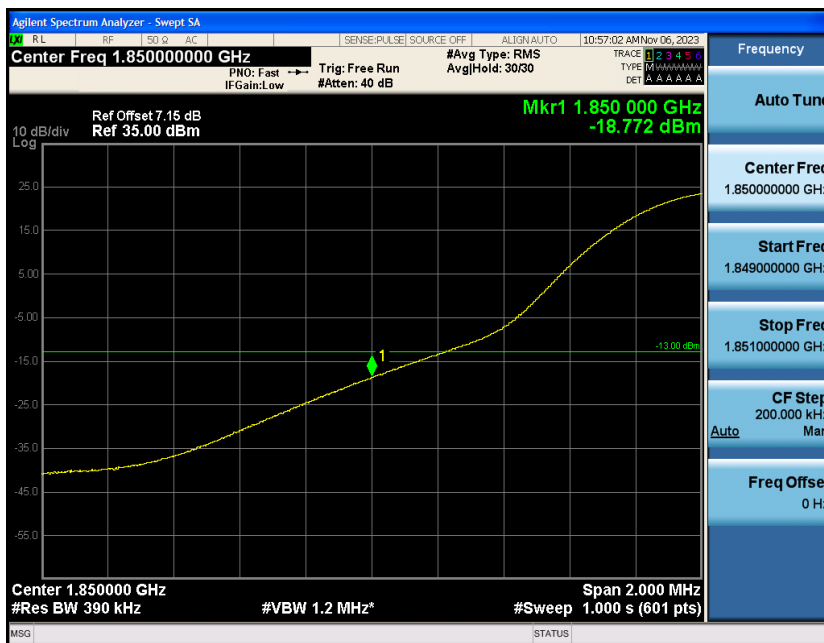
Band2-20MHz-QPSK-18700-1RB#99
