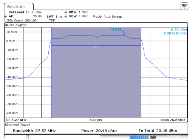
MIMO B-802.11ax/be-40MHz-Ch54-5270MHz-MCS0
