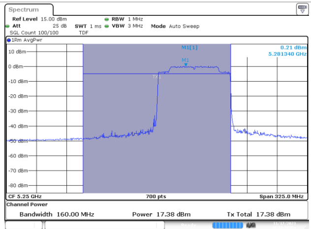
MIMO B-802.11ax/be-160MHz-Ch50-5250MHz-MCS0 80m/S67
