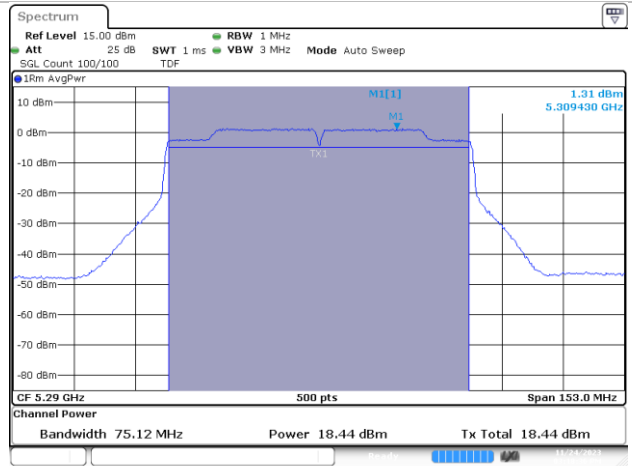
MIMO B-802.11ac-80MHz-Ch58-5290MHz-VHT0
