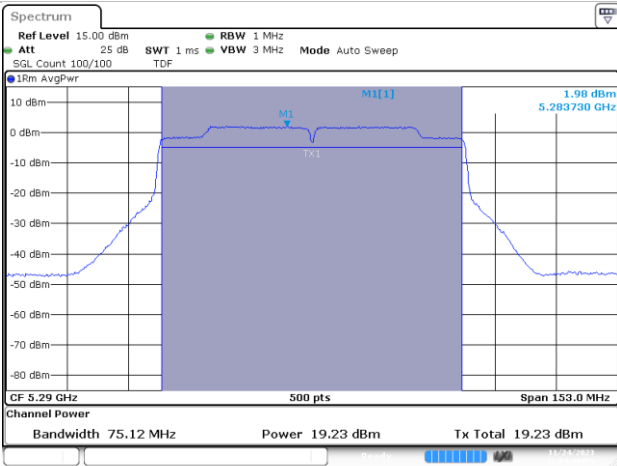
MIMO A-802.11ac-80MHz-Ch58-5290MHz-VHT0
