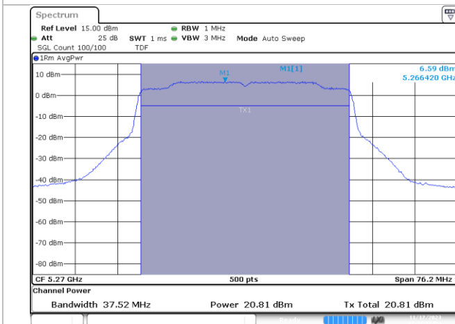
MIMO A-802.11ax/be-40MHz-Ch54-5270MHz-MCS0
