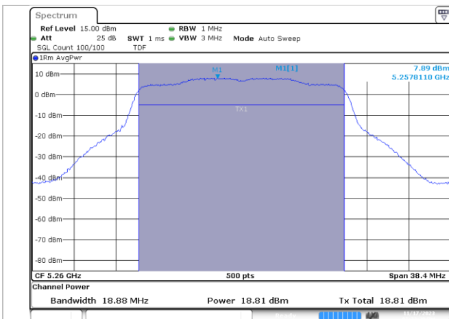
MIMO A-802.11ax/be-20MHz-Ch52-5260MHz-MCS0
