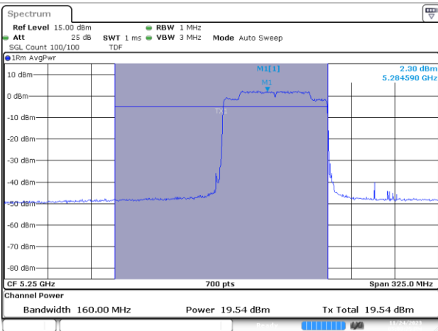
MIMO A-802.11ax/be-160MHz-Ch50-5250MHz-MCS0 80m/S67
