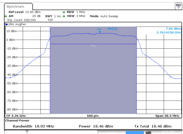
MIMO B-802.11ax/be-20MHz-Ch52-5260MHz-MCS0
