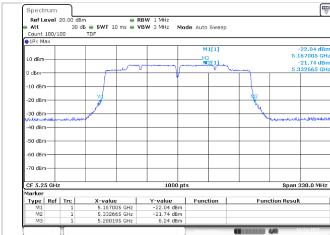
SISO B-802.11ac-160MHz-50-5250-VHT0 -26dB
