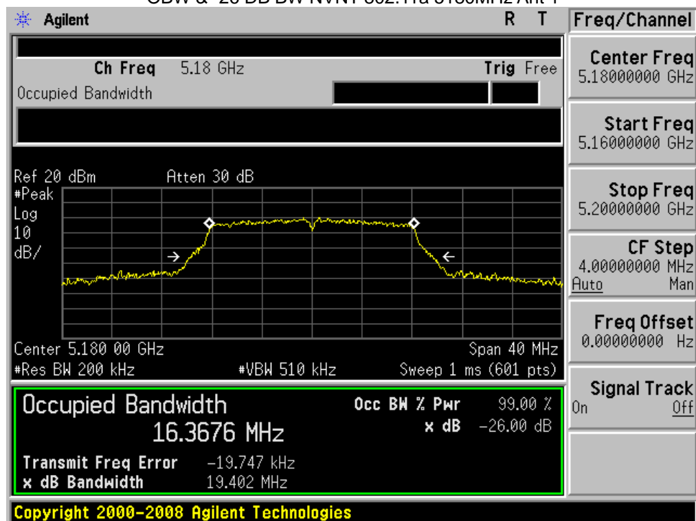
OBW & -26 DB BW NVNT 802.11a 5180MHz Ant 1
