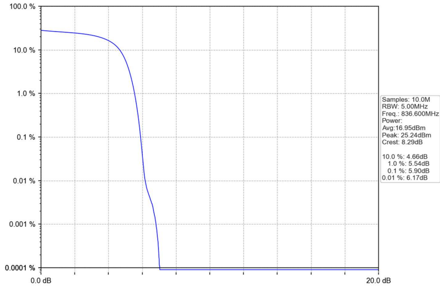
Band5_HSUPA_MCH_836.6MHz_Subtest 1_NTNV
