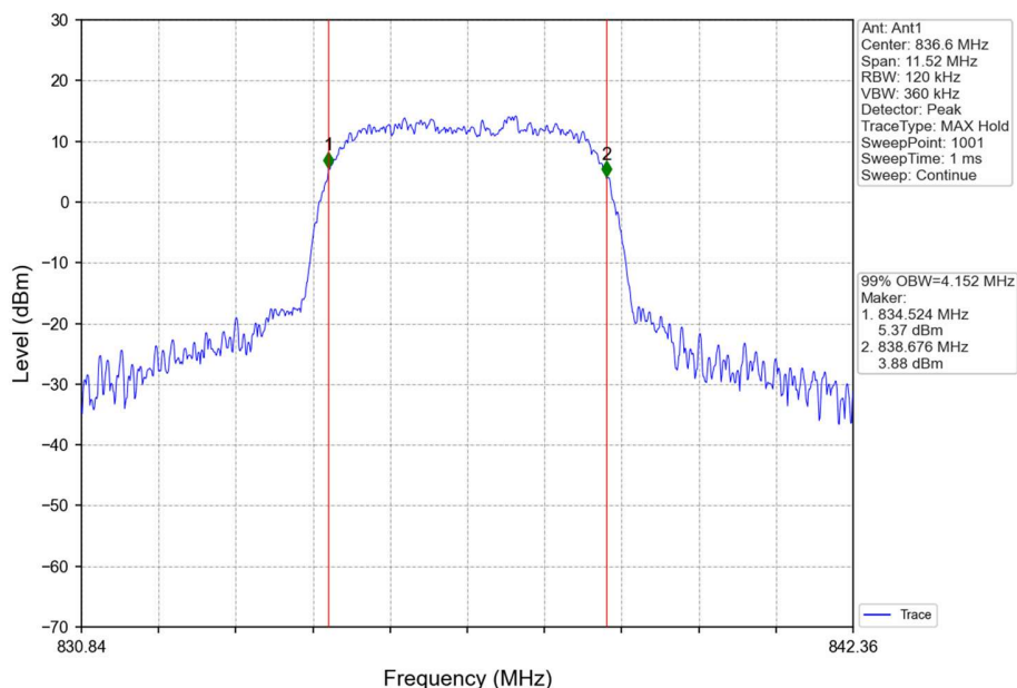
Band5_HSUPA_MCH_836.6MHz_Subtest 1_NTNV
