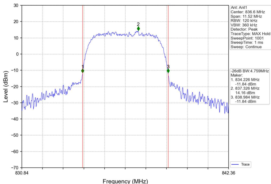
Band5_HSUPA_MCH_836.6MHz_Subtest 1_NTNV
