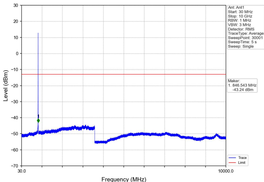
Band5_HSUPA_MCH_836.6MHz_Subtest 1_NTNV
