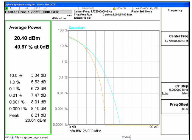
66B / 10+5MHz / High CH / 16QAM
