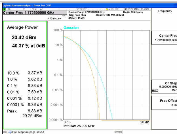
66B / 10+5MHz / High CH / 64QAM
