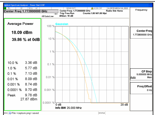
66B / 5+10MHz / High CH / 256QAM
