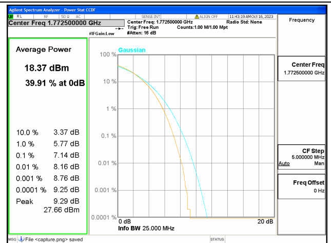
66B / 10+5MHz / High CH / 256QAM
