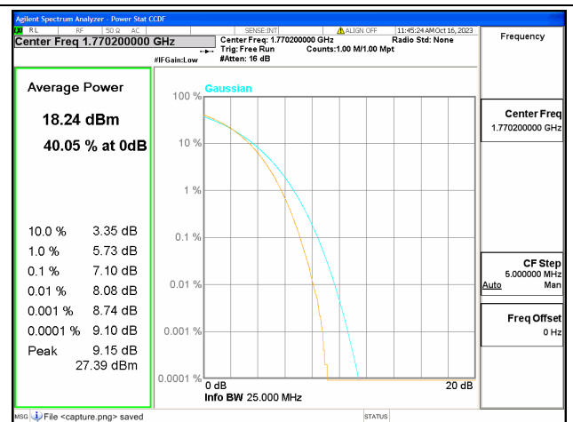
66B / 15+5MHz / High CH / 256QAM
