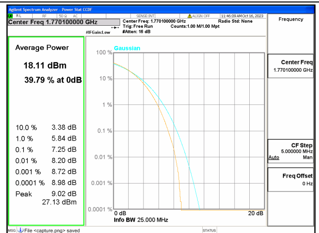
66B / 10+10MHz / High CH / 256QAM
