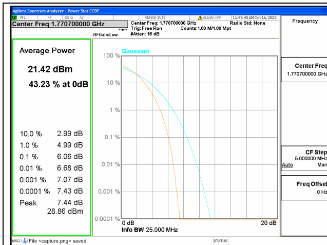
66B / 5+15MHz / High CH / QPSK
