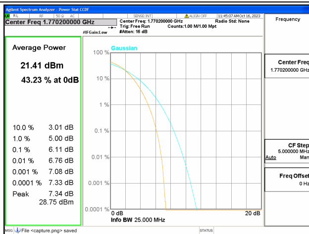
66B / 15+5MHz / High CH / QPSK
