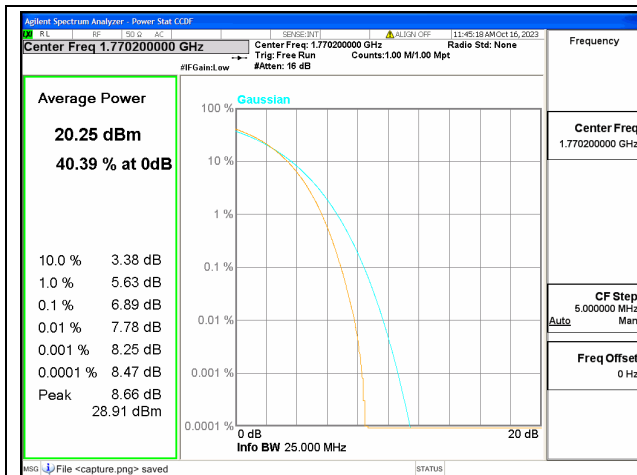
66B / 15+5MHz / High CH / 64QAM
