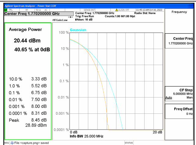
66B / 15+5MHz / High CH / 16QAM
