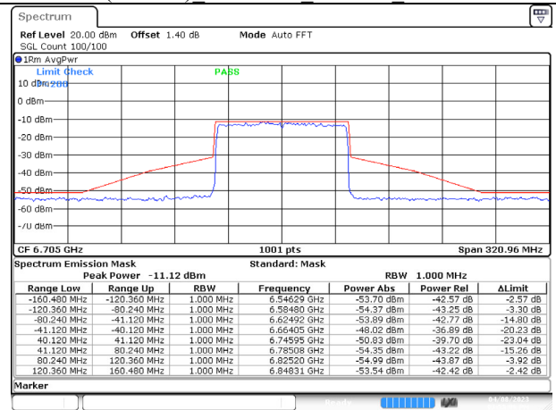
802.11ax (80MHz) 6705MHz Chain B NSS-1
