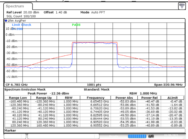
802.11ax (80MHz) 6785MHz Chain B NSS-1
