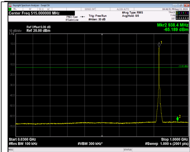
5-5-3MHz-5MHz-QPSK-QPSK-20501-20540-15RB#0-25 RB#0-30~1000MHz-PASS
