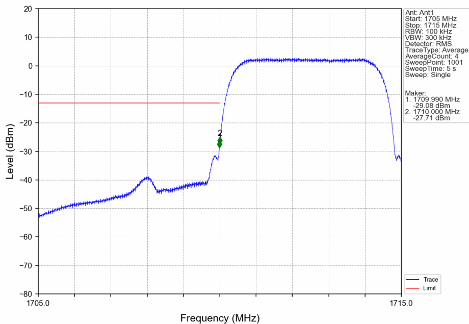
Band4_HSUPA_LCH_1712.4MHz_Subtest 1_NTNV
