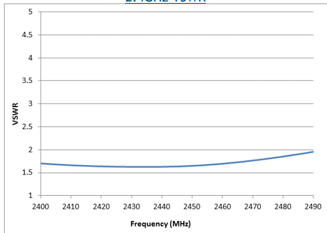
2.4GHz VSWR
