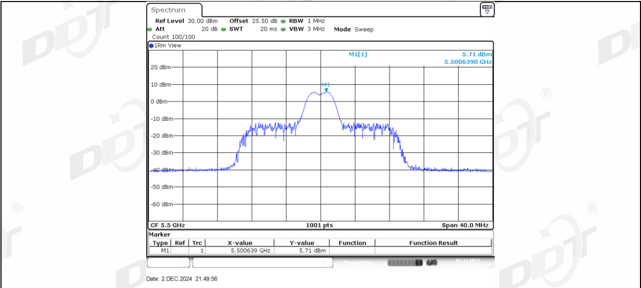
11AX20MIMO_Ant1_5500_26Tone_RU8
