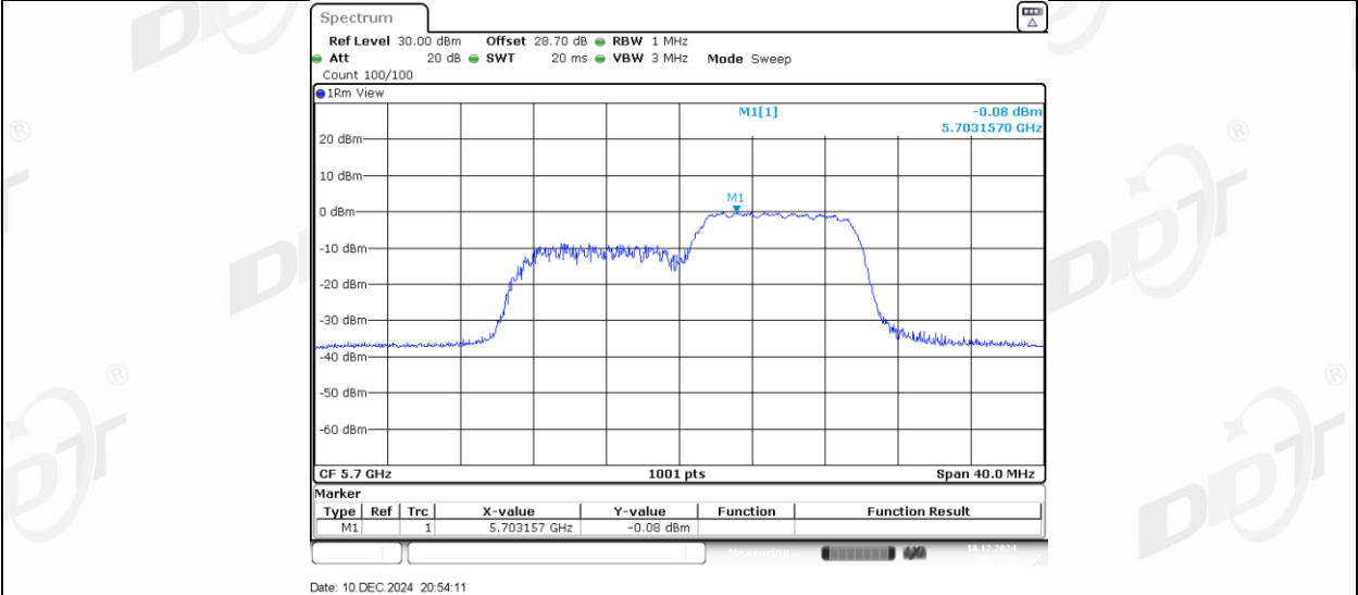
11AX20MIMO_Ant2_5700_26Tone_RU0
