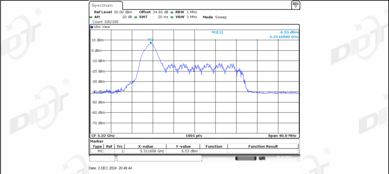
11AX20MIMO_Ant1_5320_26Tone_RU4
