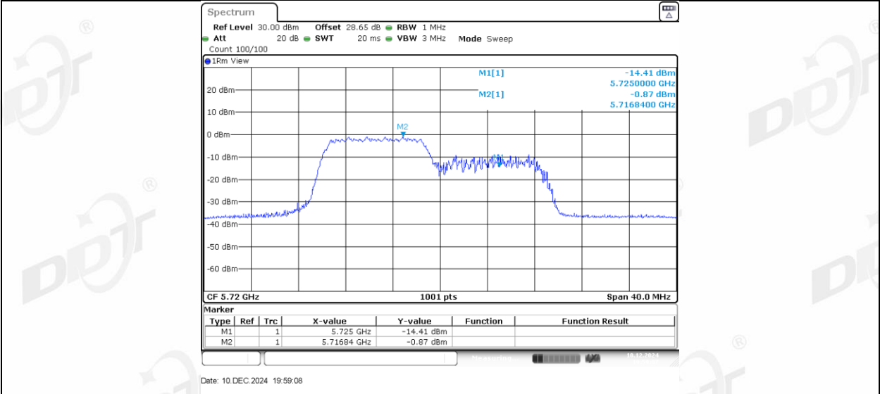
11AX20MIMO_Ant2_5720_UNII-2C_106Tone_RU54
