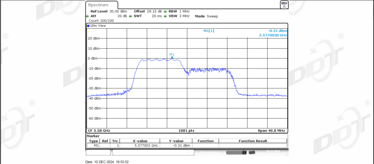
11AX20MIMO_Ant2_5580_106Tone_RU54
