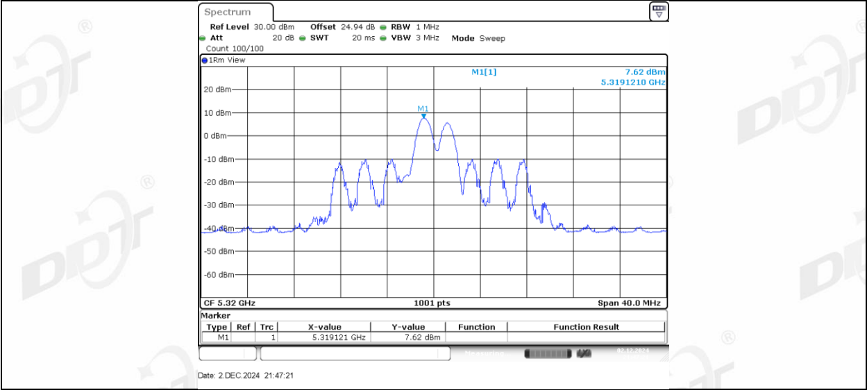
11AX20MIMO_Ant2_5320_26Tone_RU8
