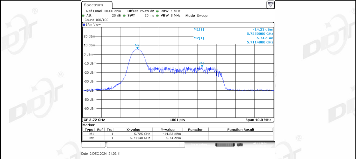
11AX20MIMO_Ant2_5720_UNII-2C_26Tone_RU4
