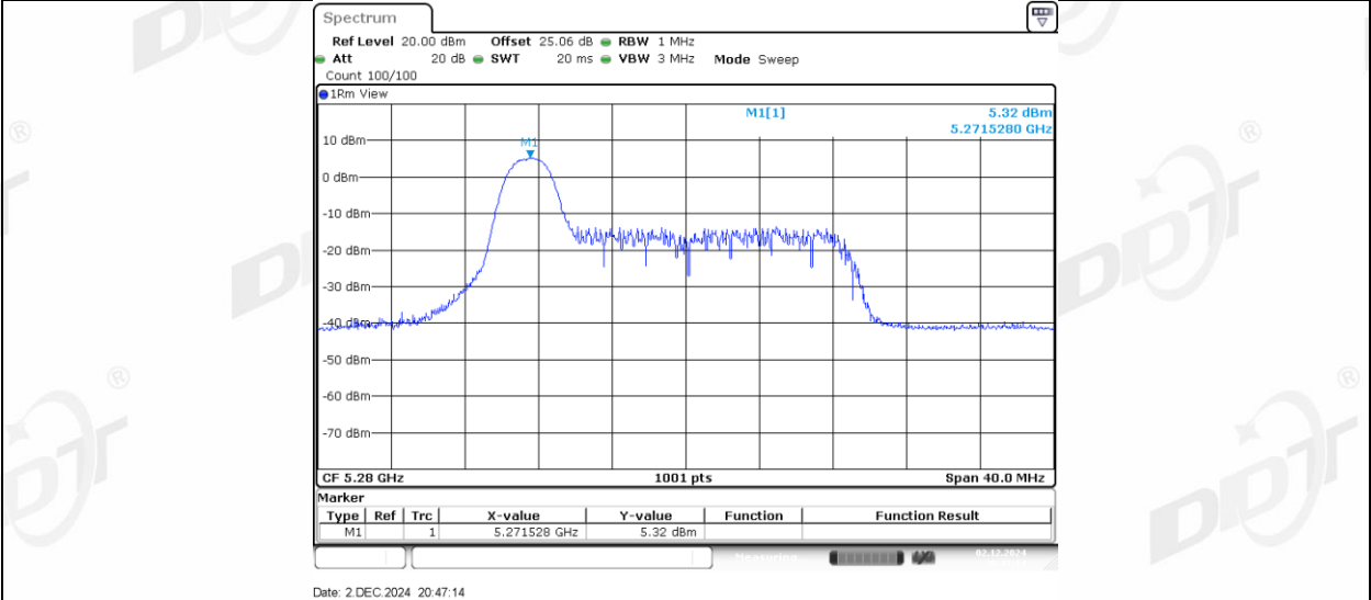
11AX20MIMO_Ant2_5280_26Tone_RU4
