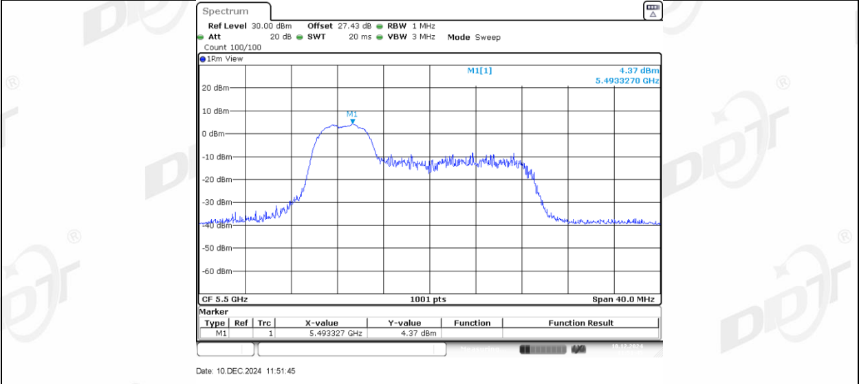
11AX20MIMO_Ant1_5500_52Tone_RU39
