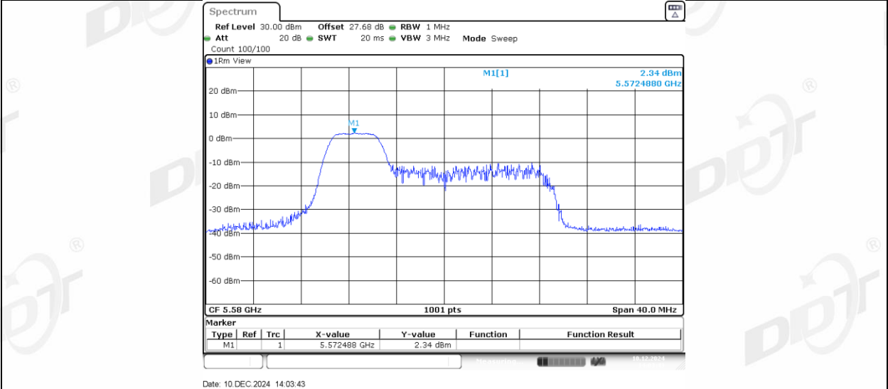
11AX20MIMO_Ant2_5580_52Tone_RU39
