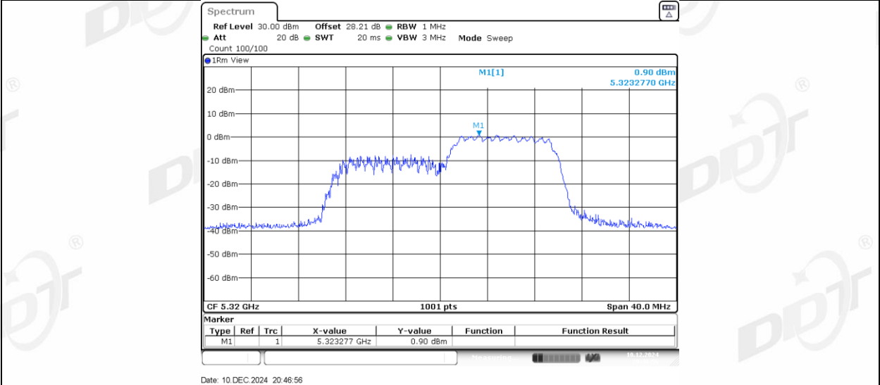
11AX20MIMO_Ant2_5320_26Tone_RU0
