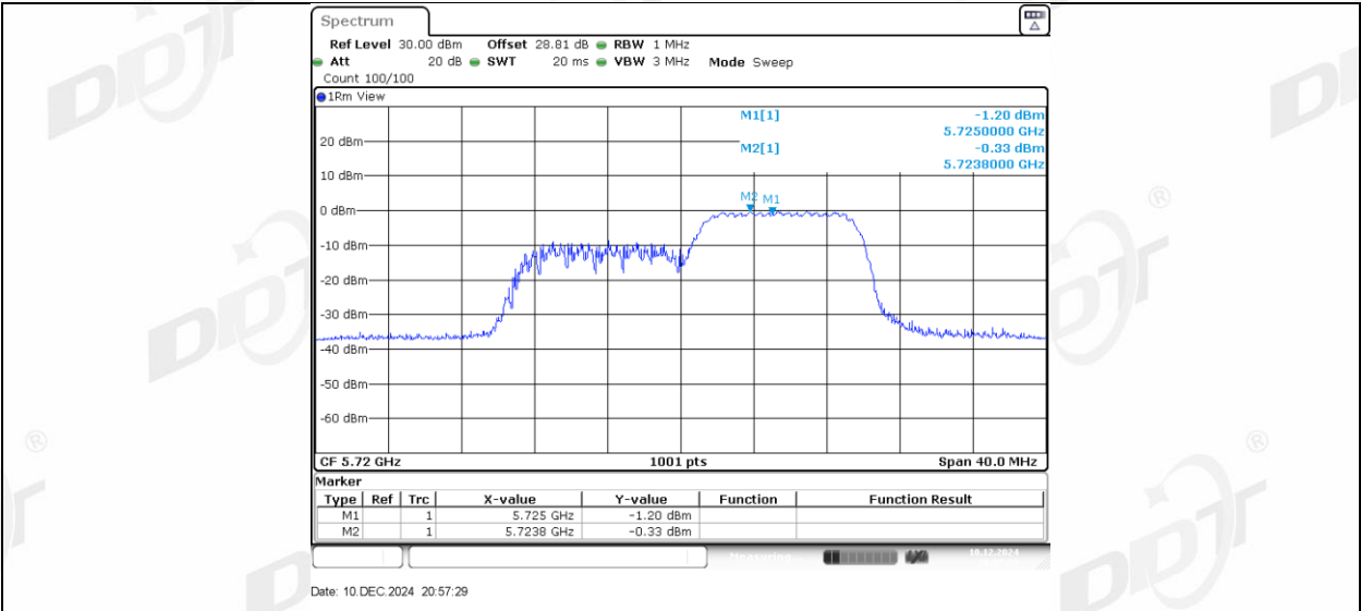
11AX20MIMO_Ant2_5720_UNII-2C_26Tone_RU0
