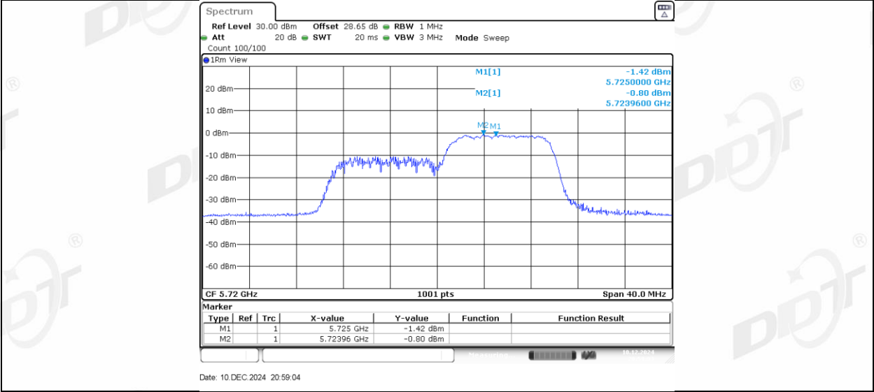
11AX20MIMO_Ant1_5720_UNII-3_26Tone_RU0
