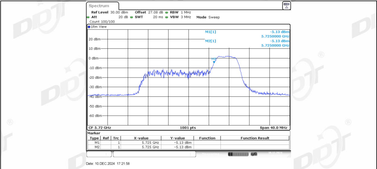
11AX20MIMO_Ant2_5720_UNII-2C_106Tone_RU53
