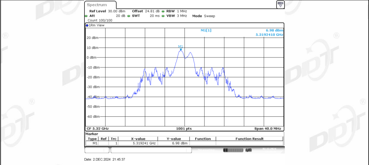
11AX20MIMO_Ant1_5320_26Tone_RU8
