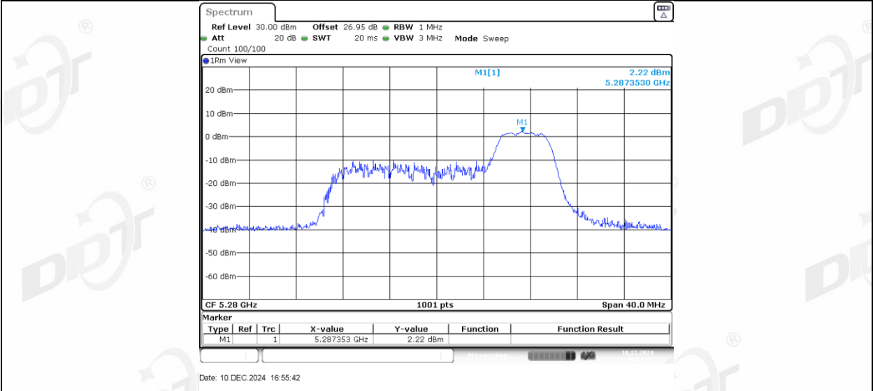
11AX20MIMO_Ant2_5280_106Tone_RU53
