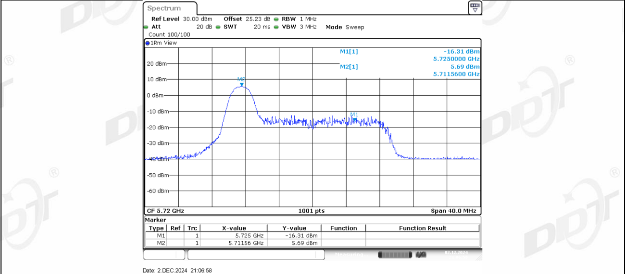
11AX20MIMO_Ant1_5720_UNII-2C_26Tone_RU4
