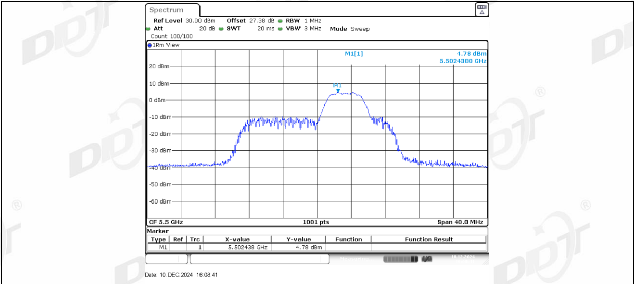
11AX20MIMO_Ant1_5500_52Tone_RU40
