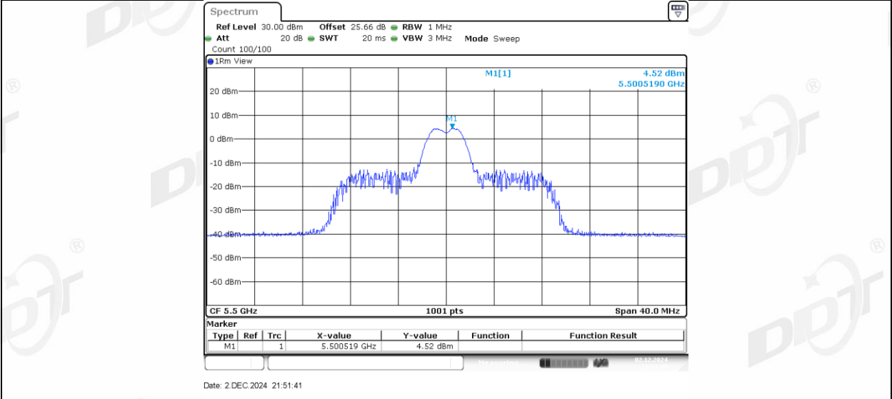
11AX20MIMO_Ant2_5500_26Tone_RU8
