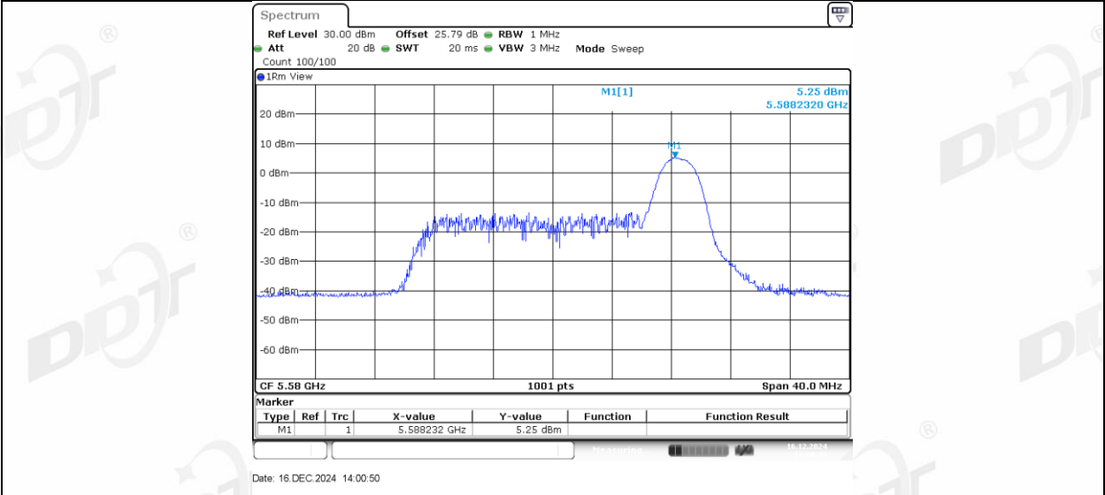
11AX20MIMO_Ant2_5580_52Tone_RU37
