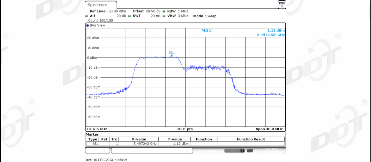
11AX20MIMO_Ant1_5500_106Tone_RU54
