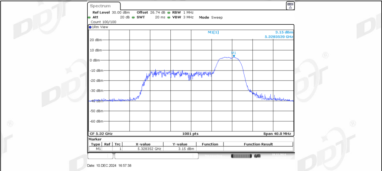
11AX20MIMO_Ant1_5320_106Tone_RU53
