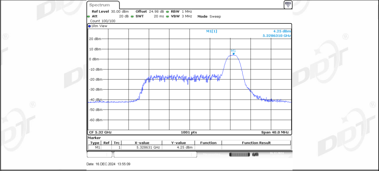
11AX20MIMO_Ant2_5320_52Tone_RU37
