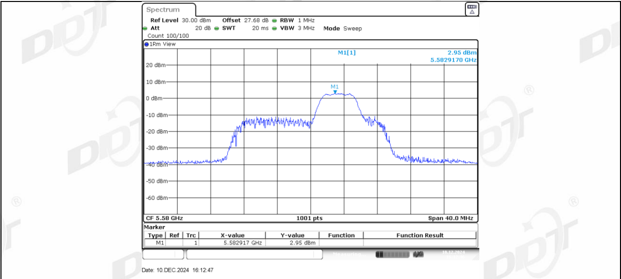
11AX20MIMO_Ant2_5580_52Tone_RU40
