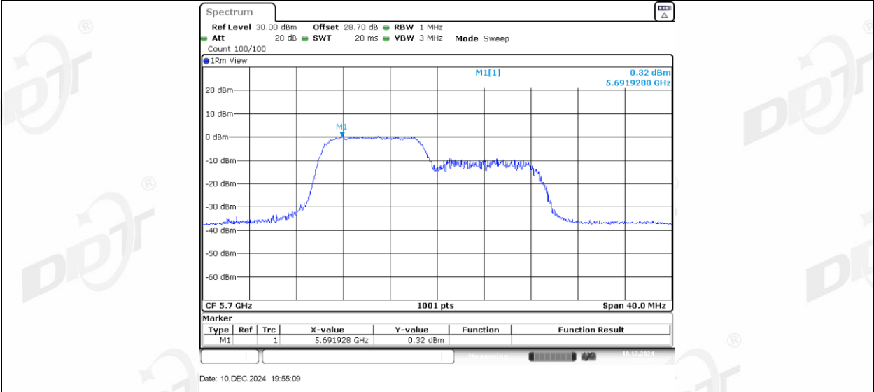
11AX20MIMO_Ant1_5700_106Tone_RU54
