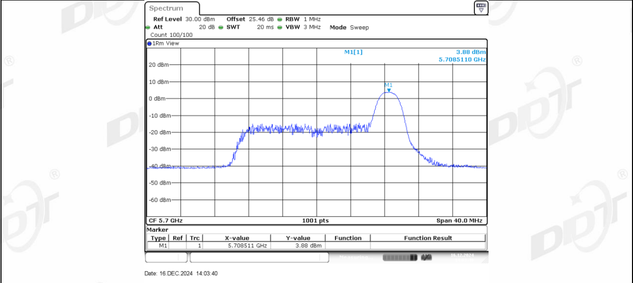
11AX20MIMO_Ant2_5700_52Tone_RU37
