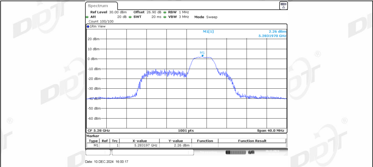
11AX20MIMO_Ant2_5280_52Tone_RU40
