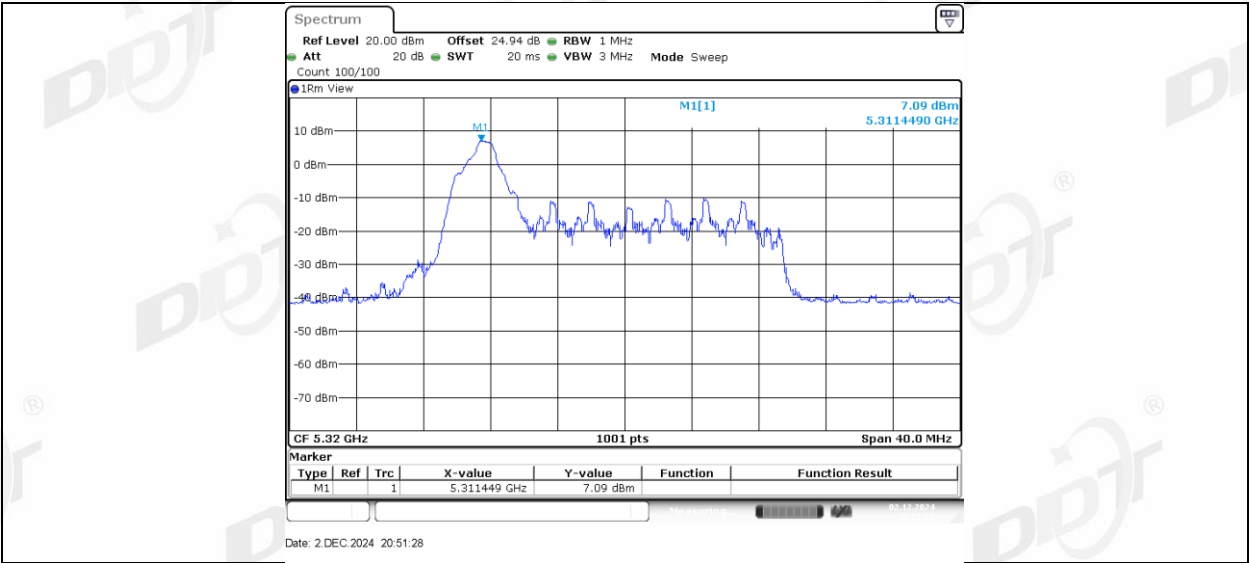
11AX20MIMO_Ant2_5320_26Tone_RU4
