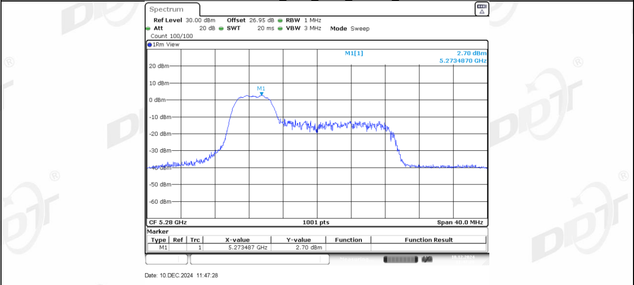
11AX20MIMO_Ant2_5280_52Tone_RU39
