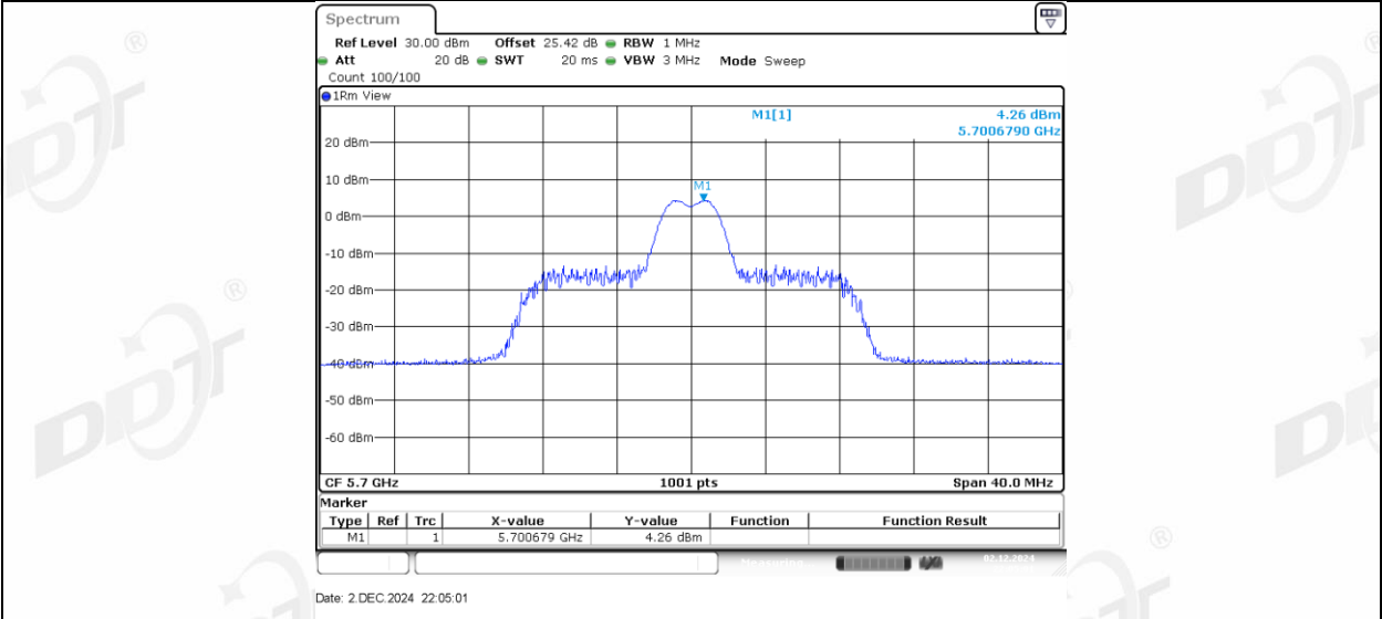
11AX20MIMO_Ant2_5700_26Tone_RU8
