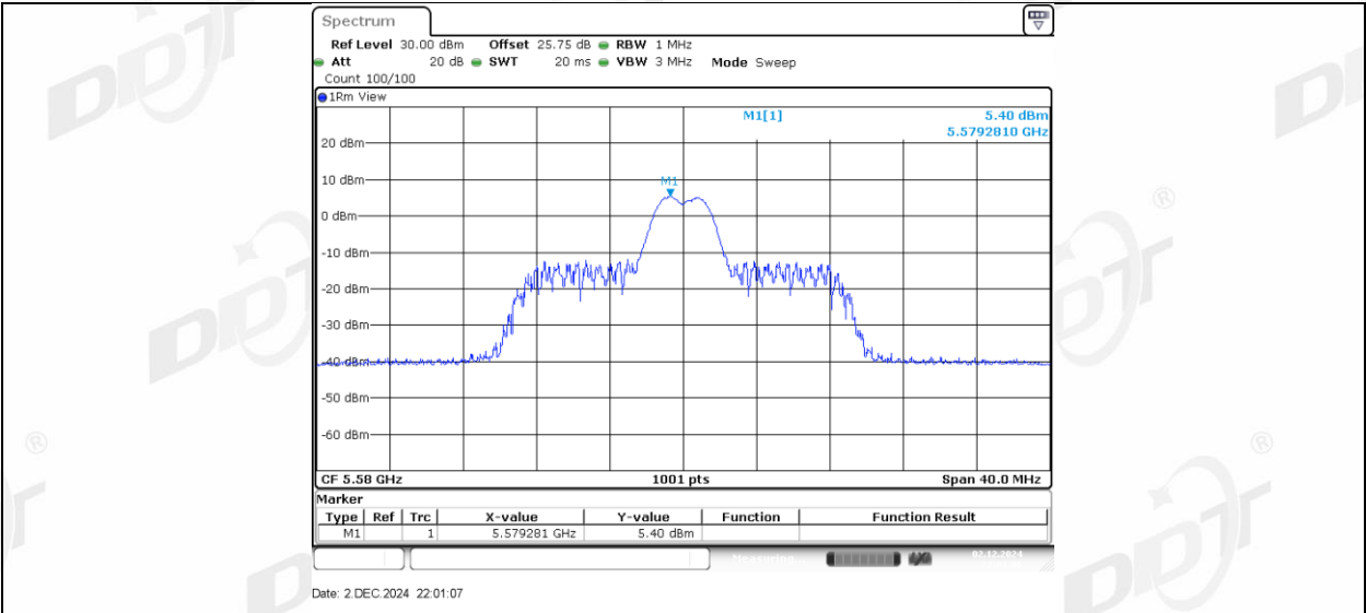
11AX20MIMO_Ant2_5580_26Tone_RU8
