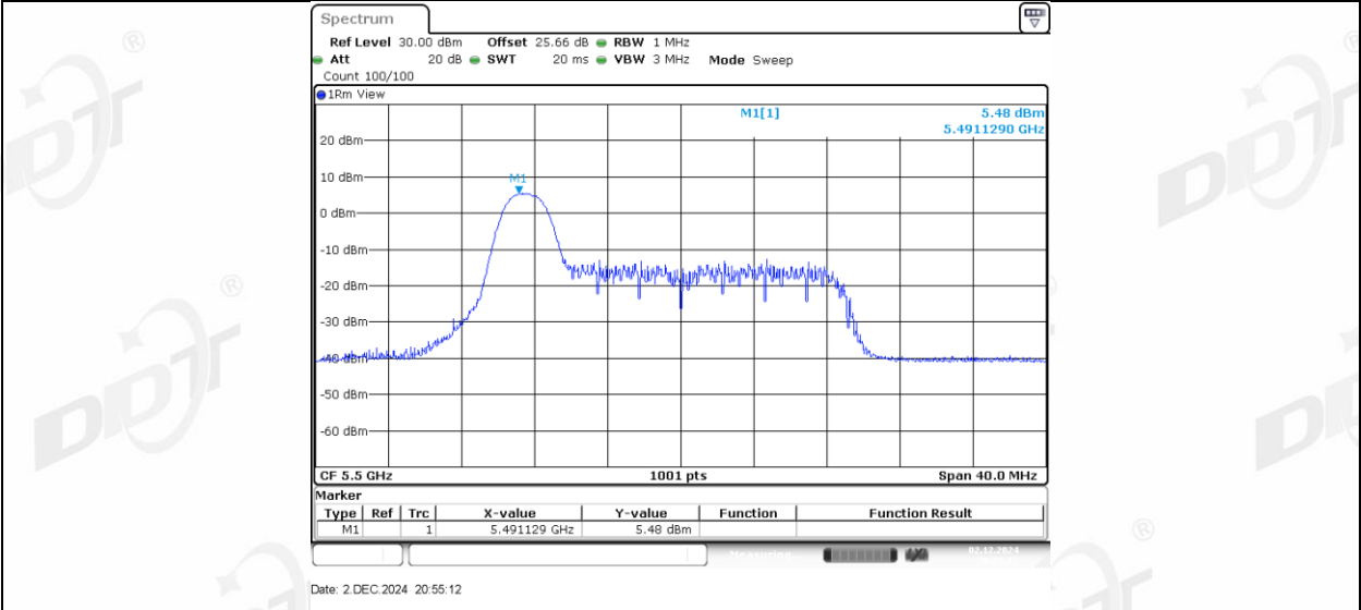
11AX20MIMO_Ant2_5500_26Tone_RU4
