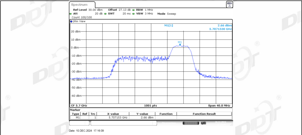
11AX20MIMO_Ant1_5700_106Tone_RU53
