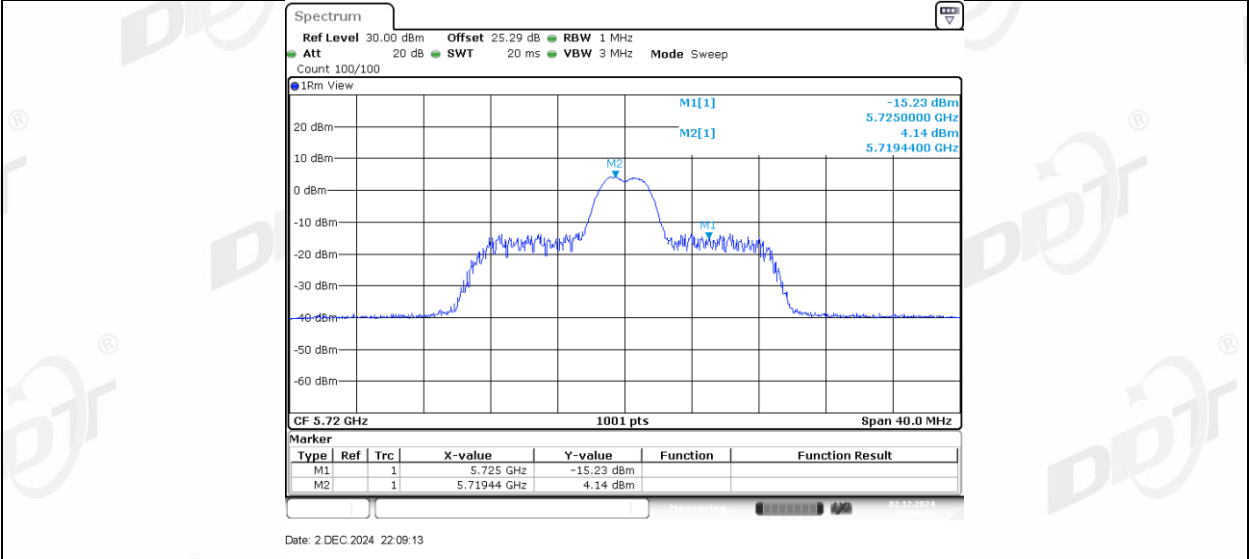
11AX20MIMO_Ant2_5720_UNII-2C_26Tone_RU8
