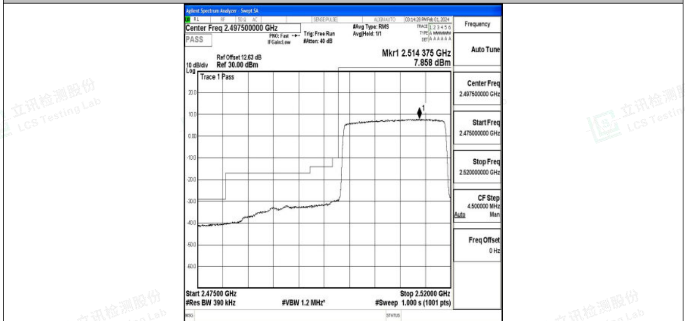
Band7_20MHz_QPSK_20850_100RB#0
