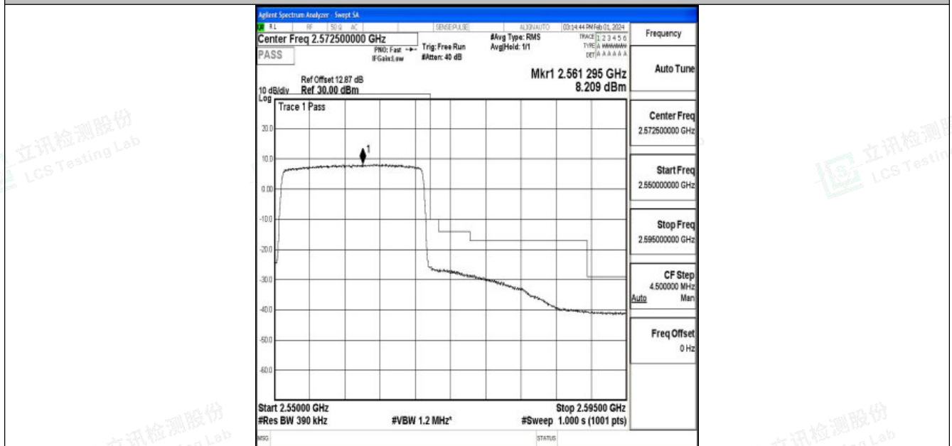
Band7_20MHz_QPSK_21350_100RB#0
