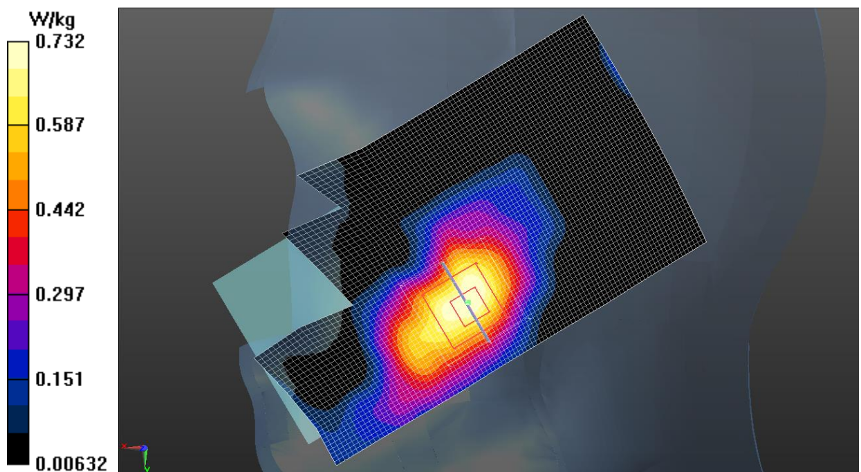
Fig.7 CDMA BC1
