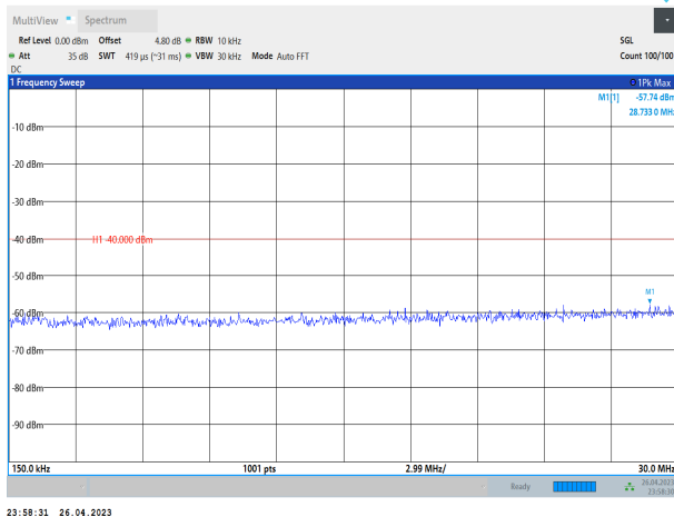
Band30-10MHz-QPSK-27710-1RB#0-Range2:0.15~30MHz
