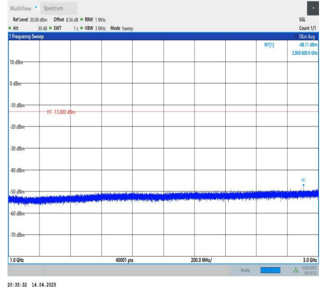
Band26(824-849)-3MHz-QPSK-26805-1RB#0-1000~3000-PASS
