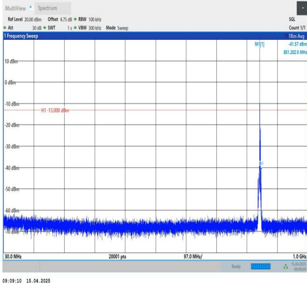
Band26(824-849)-3MHz-QPSK-27025-1RB#0-30~1000-PASS
