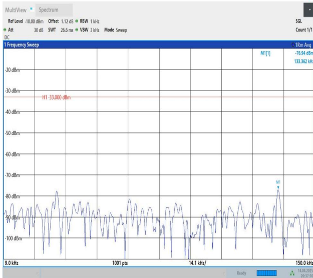
Band26(824-849)-3MHz-QPSK-27025-1RB#0-0.009~0.15-PASS
