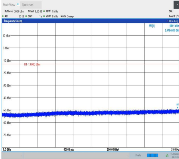
Band26(824-849)-3MHz-QPSK-26915-1RB#14-1000~3000-PASS
