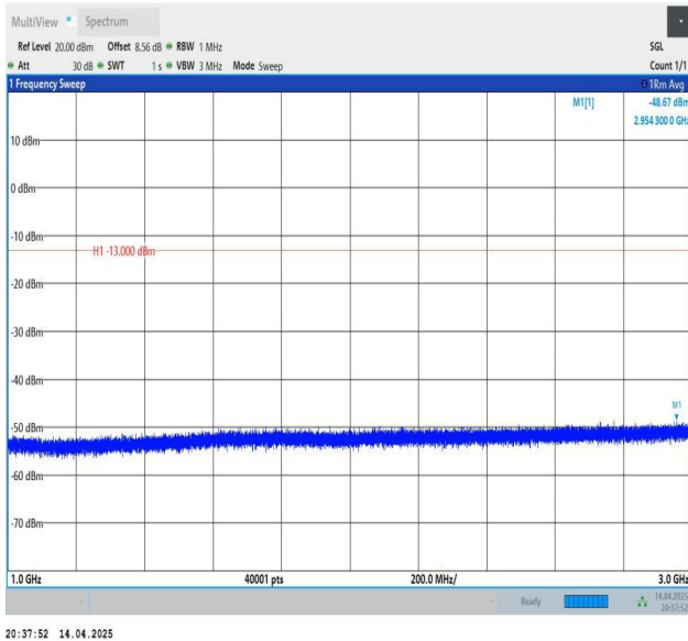
Band26(824-849)-3MHz-QPSK-27025-1RB#14-1000~3000-PASS
