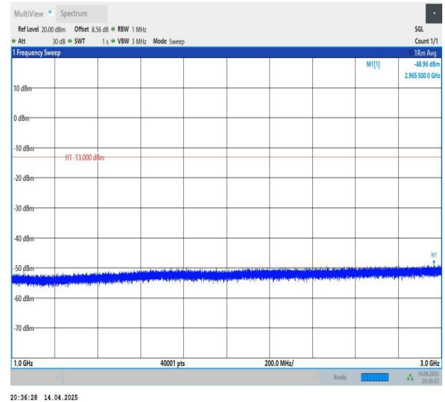
Band26(824-849)-3MHz-QPSK-26915-1RB#0-1000~3000-PASS
