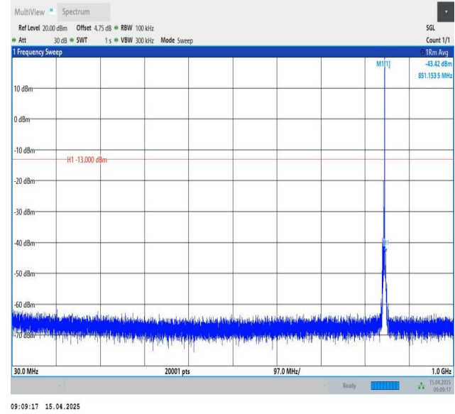
Band26(824-849)-3MHz-QPSK-27025-1RB#14-30~1000-PASS
