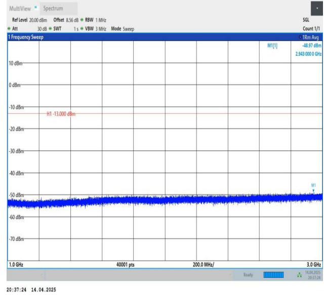
Band26(824-849)-3MHz-QPSK-27025-1RB#0-1000~3000-PASS
