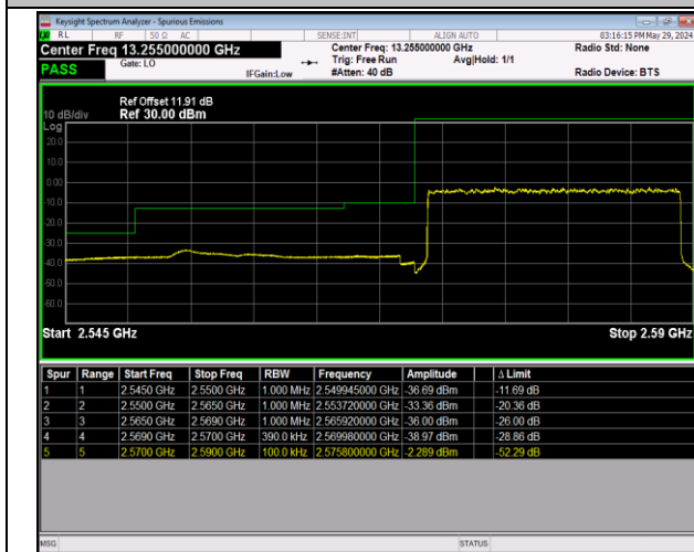
Band38_20MHz_QPSK_37850_100RB#0
