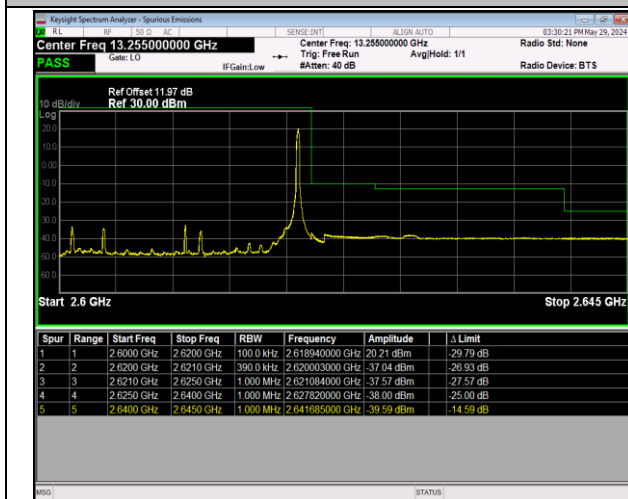
Band38_20MHz_QPSK_38150_1RB#99
