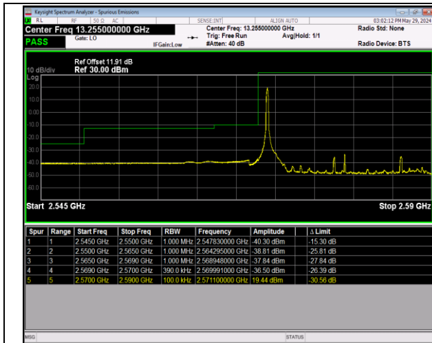
Band38_20MHz_QPSK_37850_1RB#0
