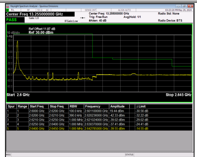
Band38_20MHz_QPSK_38150_1RB#0
