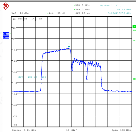
11AX80SISO-Ant1-5210-484Tone-RU65-PASS
