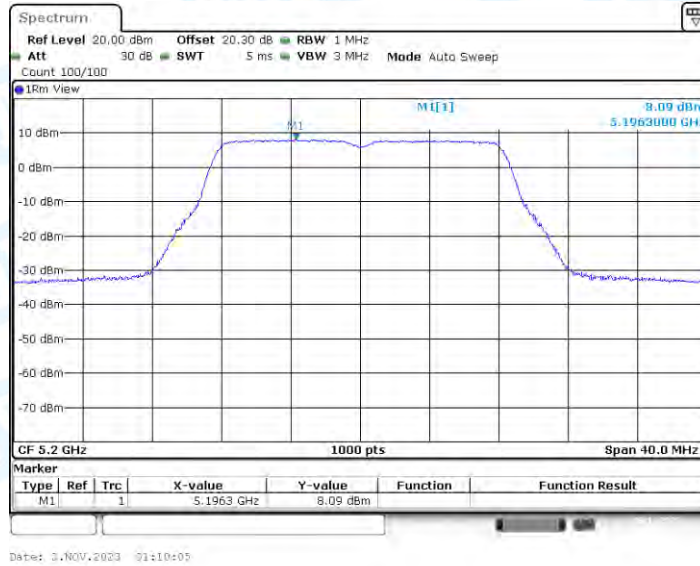
11A-CDD_Ant3_5200
