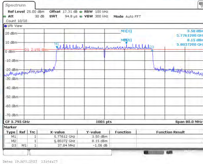
11AX40-CDD_Ant2_5795
