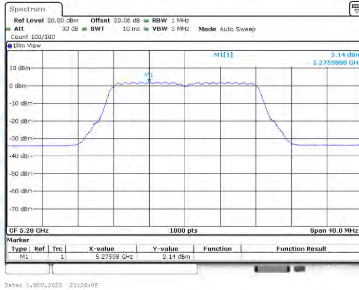
11A-CDD_Ant3_5280
