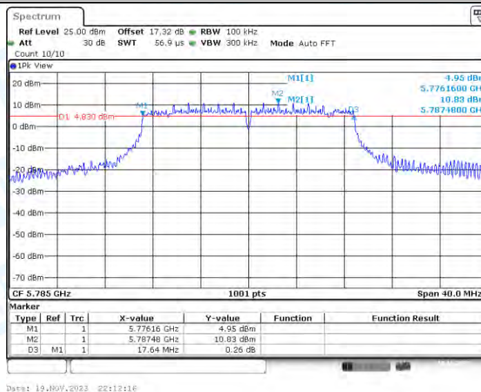
11N20-CDD_Ant3_5785
