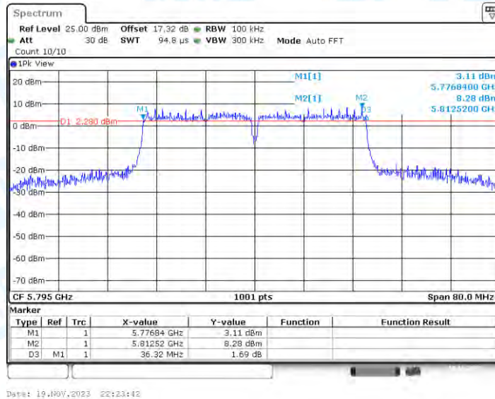
11N40-CDD_Ant3_5795
