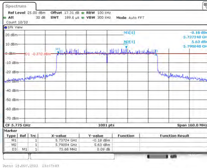
11AX80-CDD_Ant2_5775
