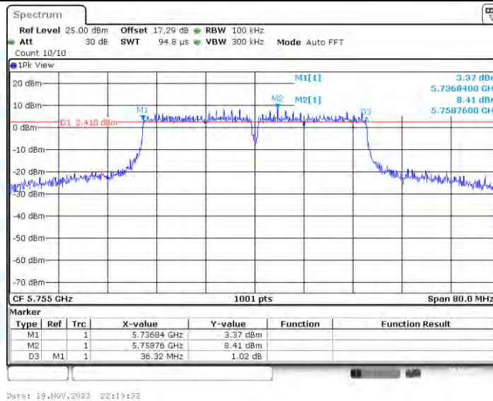
11N40-CDD_Ant3_5755
