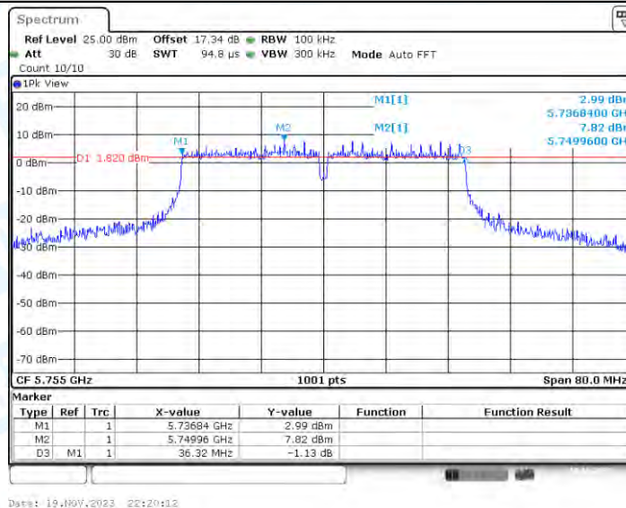
11N40-CDD_Ant4_5755
