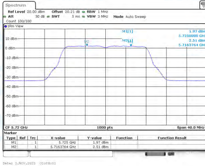
11A-CDD_Ant3_5720_UNII-2C
