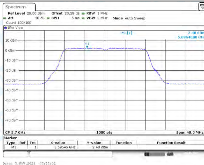
11A-CDD_Ant3_5700
