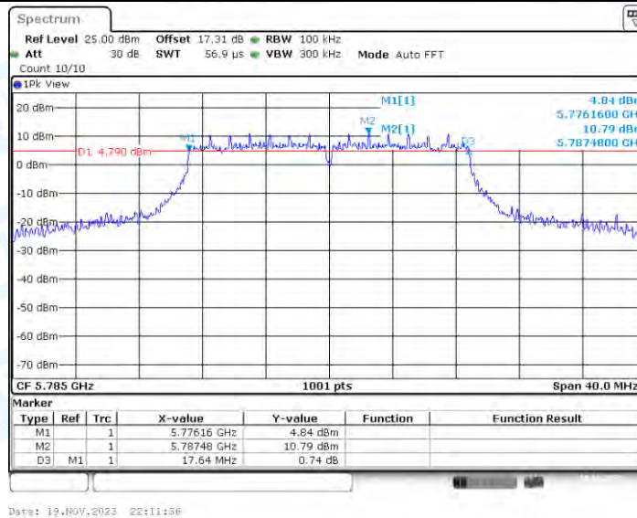
11N20-CDD_Ant2_5785
