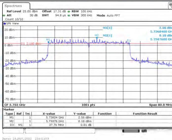
11AX40-CDD_Ant2_5755
