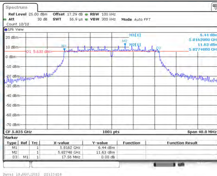
11N20-CDD_Ant2_5825
