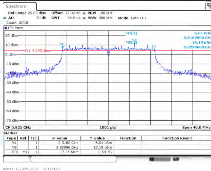
11N20-CDD_Ant4_5825
