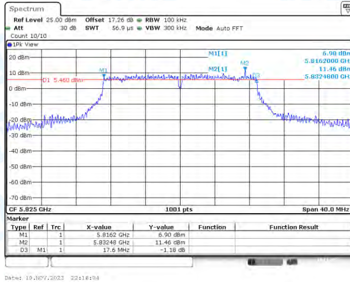
11N20-CDD_Ant3_5825
