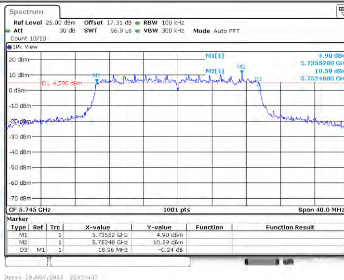
11AX20-CDD_Ant2_5745
