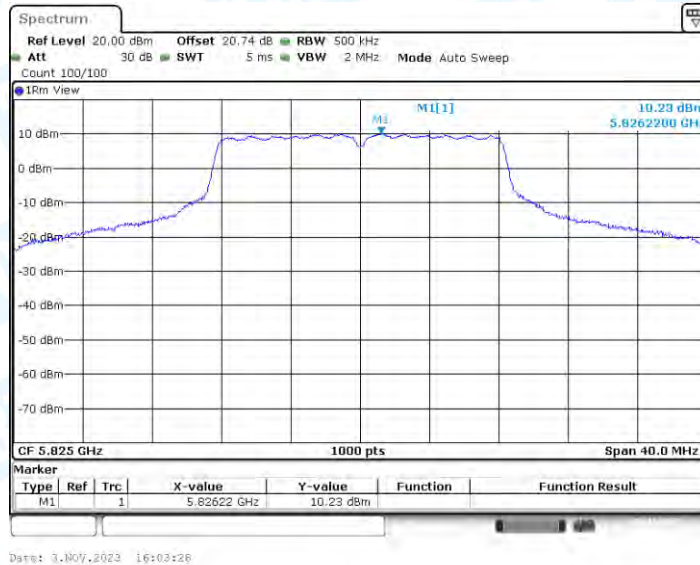
11A_Ant3_5825
