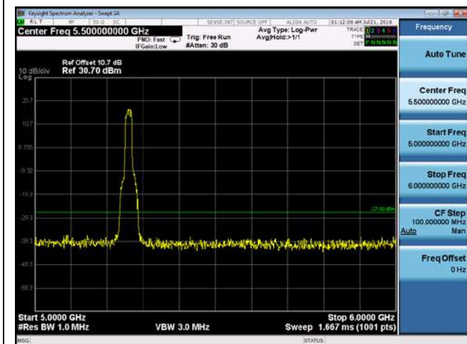
CUE-802.11n-20-5260M chain3(5GHz-6GHz)
