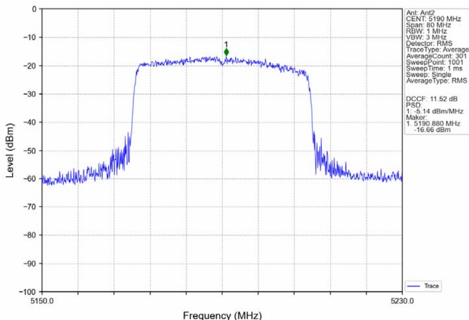
802.11ax(HEW40)_LCH_5190MHz_RU484_Left_Ant2_NTNV
