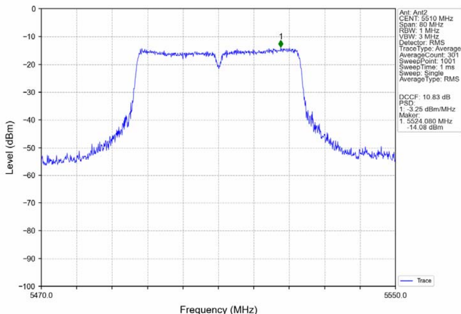
802.11n(HT40)_LCH_5510MHz_Ant2_NTNV
