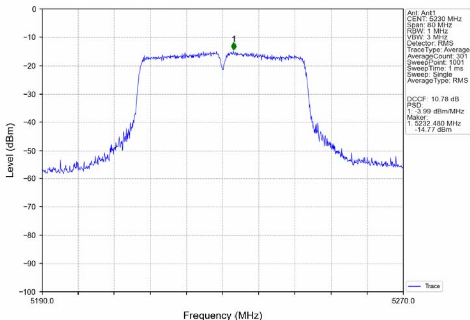
802.11n(HT40)_HCH_5230MHz_Ant1_NTNV
