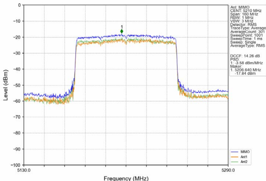
802.11ax(HEW80)_MCH_5210MHz_RU996_Left_MIMO_NTNV
