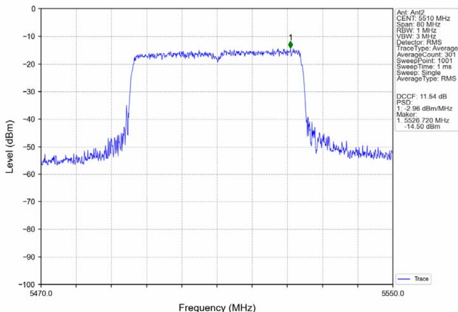
802.11ax(HEW40)_LCH_5510MHz_RU484_Left_Ant2_NTNV
