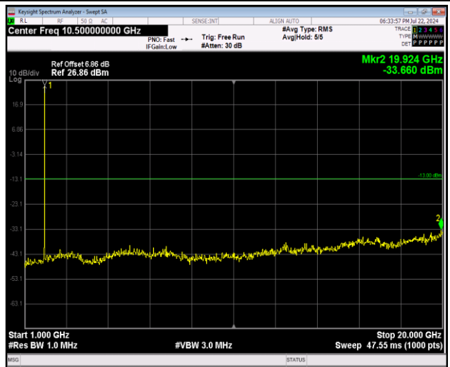
Band2-20MHz-QPSK-18700-1RB#0-Range2:1000~20000MHz
