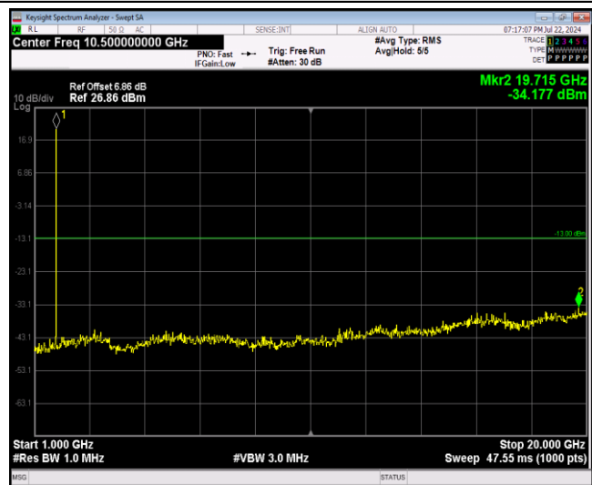
Band4-20MHz-QPSK-20050-1RB#0-Range2:1000~200 00MHz
