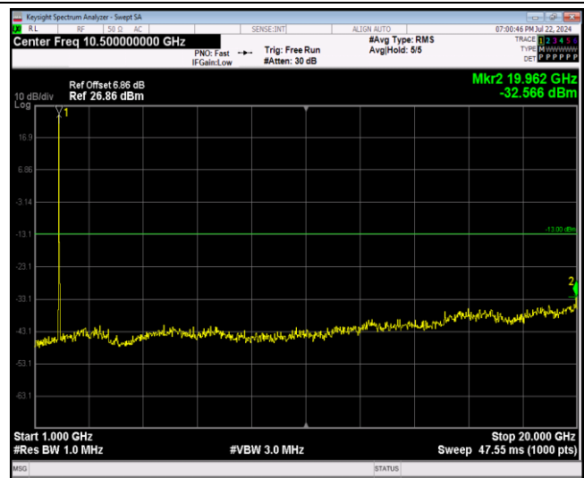
Band2-20MHz-16QAM-18900-1RB#0-Range2:1000~20000MHz
