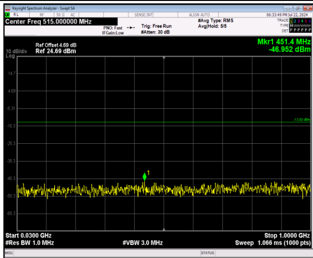
Band2-20MHz-QPSK-18700-1RB#0-Range1:30~1000MHz
