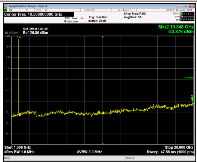
Band4-1.4MHz-QPSK-20175-1RB#0-Range2:1000~20000MHz
