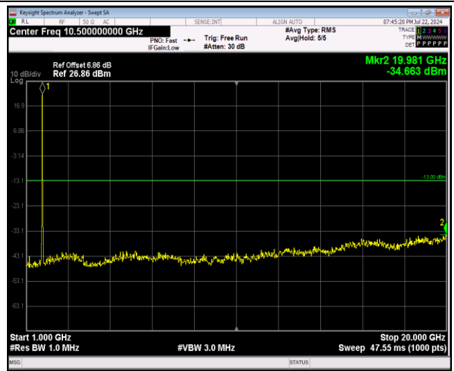
Band4-20MHz-QPSK-20300-1RB#0-Range2:1000~200 OOMHz
